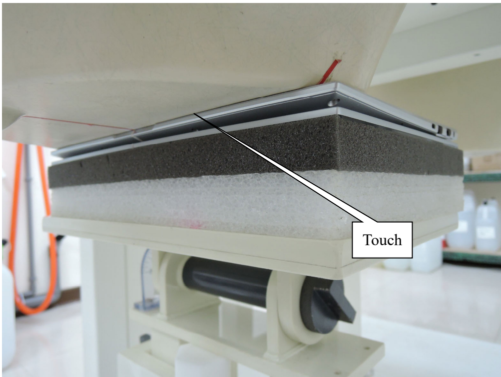
EUT Back(PAD)
