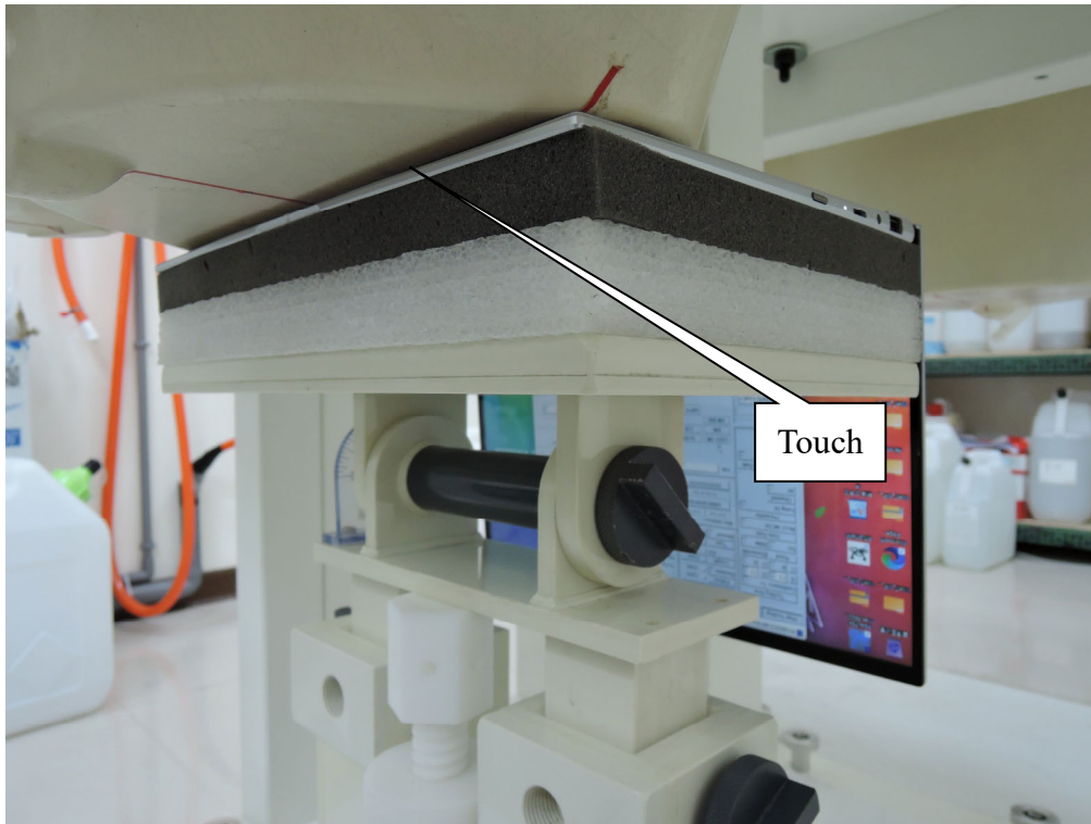
EUT Bottom(NB)
