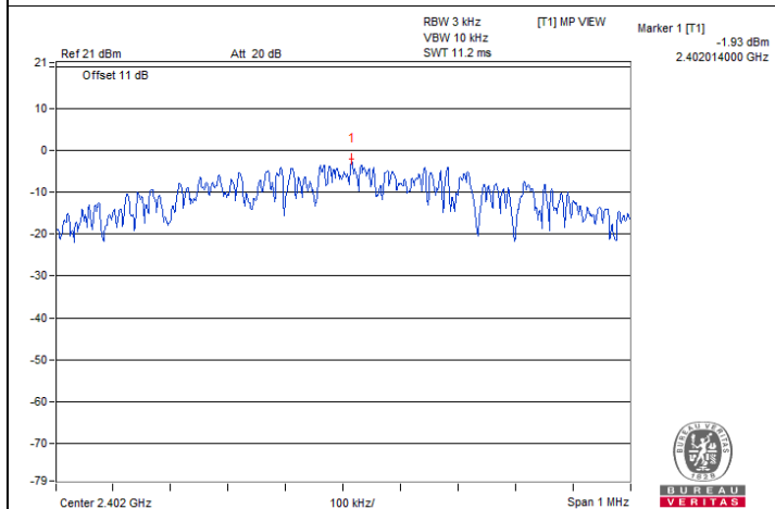
BT-LE 1M High Power : CH 0
