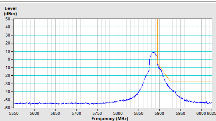
Vertical (Average)
