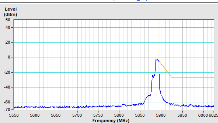
Vertical (Average)
