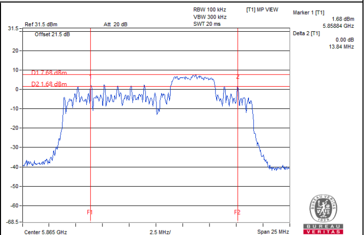
802.11ax (HE) 52-tone RU : CH 173
