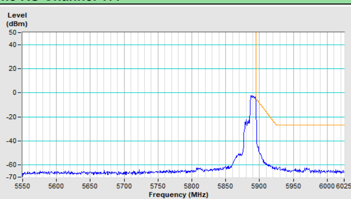
Horizontal (Average)
