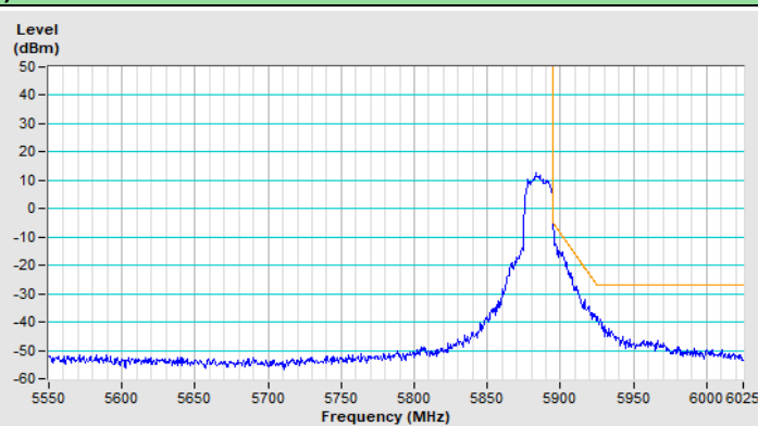
Horizontal (Average)
