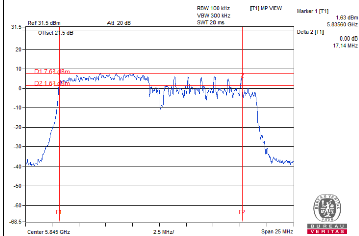
802.11ax (HE) 106-tone RU : CH 169
