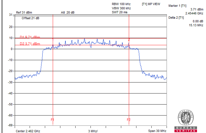
802.11ax (HE20) : CH 11
