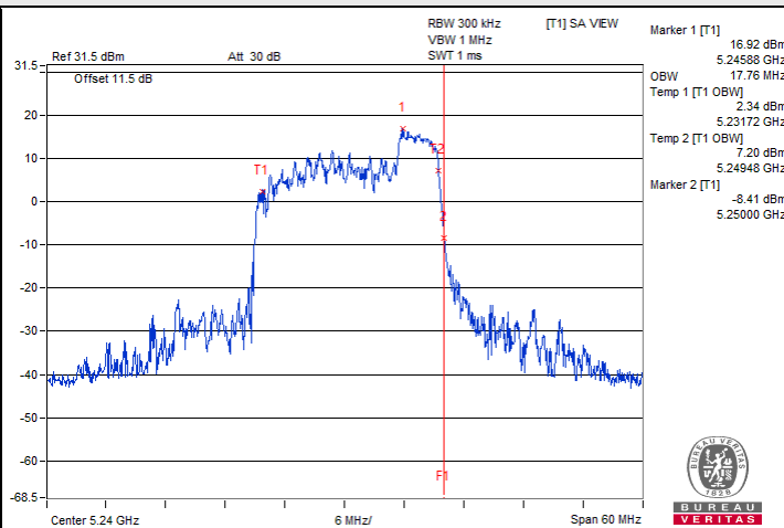
802.11ax (RU52) : CH 48
