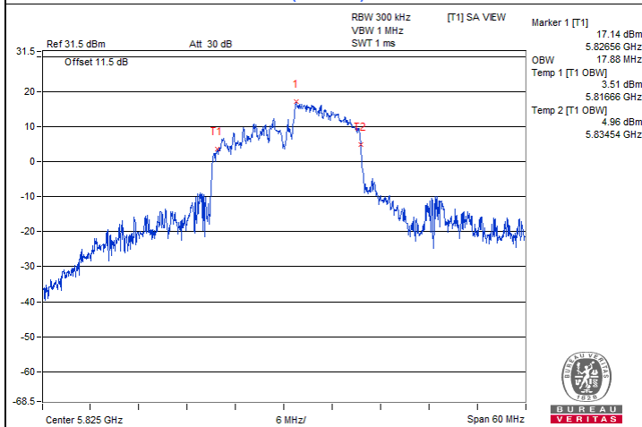
802.11ax (RU106) : CH 165
