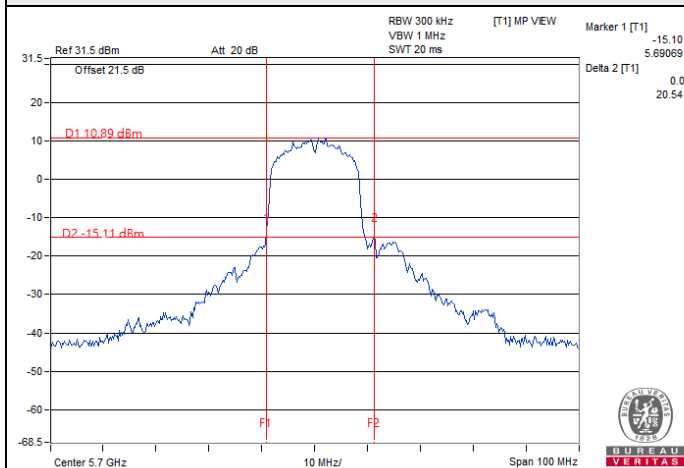
802.11a : CH 140
