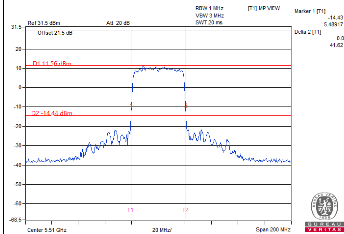
802.11ax (HE40) : CH 102
