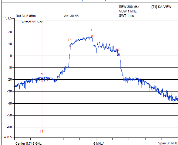
802.11ax (RU106) / Chain 0 : CH 149
