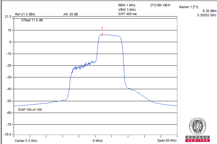
802.11ax (RU106) / Chain0 : CH 60
