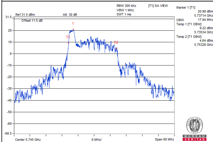
802.11ax (RU26) : CH 149
