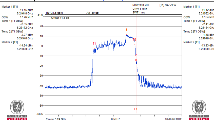
802.11ax (RU52) / Chain 1 : CH 48
