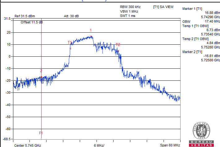
802.11ax (RU106) / Chain 1 : CH 149
