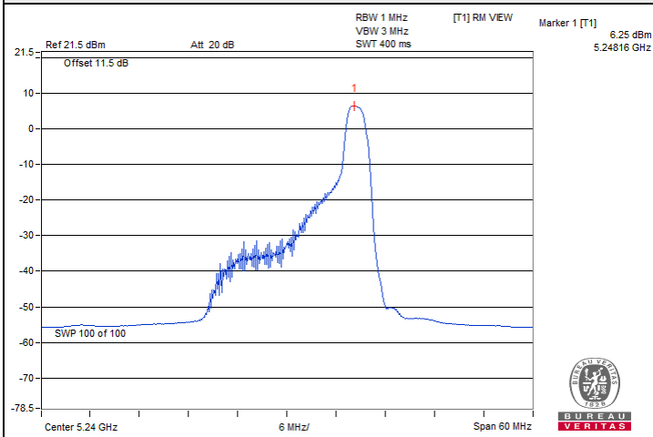
802.11ax (RU26) / Chain1 : CH 48
