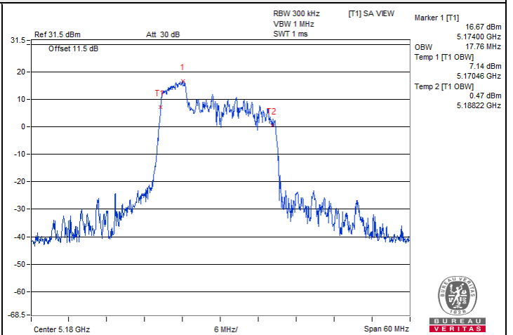
802.11ax (RU52) : CH 36
