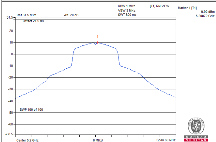
802.11a : CH 40
