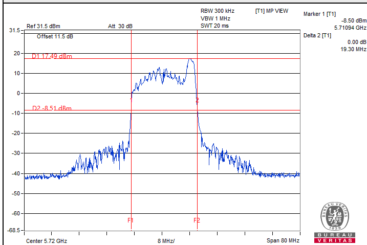
802.11ax (RU26) : CH 144 (U-NII-2C)
