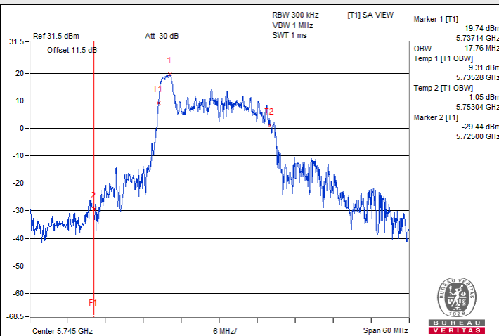
802.11ax (RU26) / Chain 1 : CH 149
