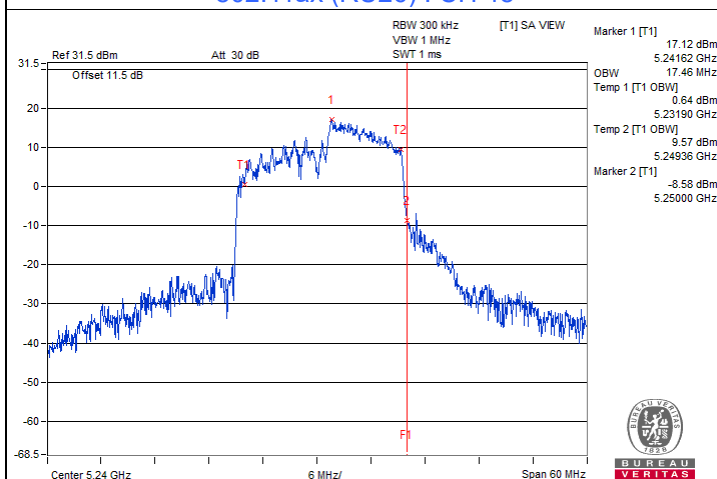
802.11ax (RU106) : CH 48
