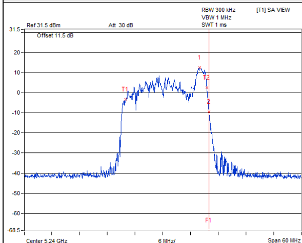
802.11ax (RU26) / Chain 0 : CH 48
