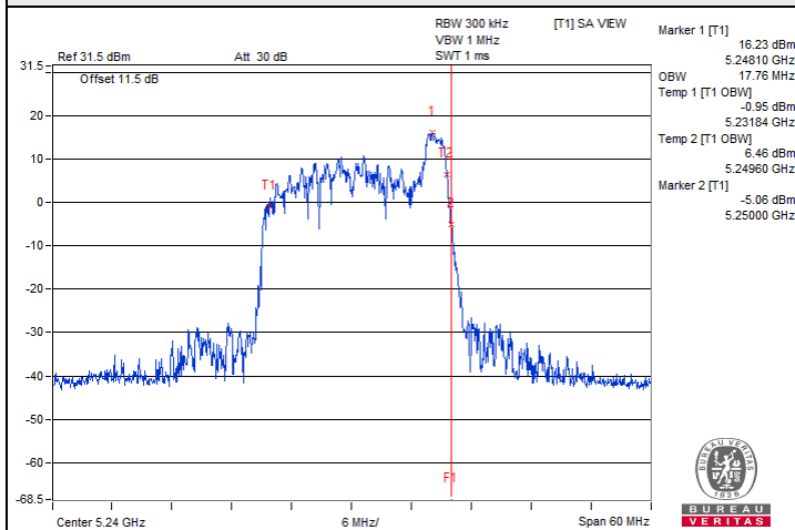
802.11ax (RU26) : CH 48
