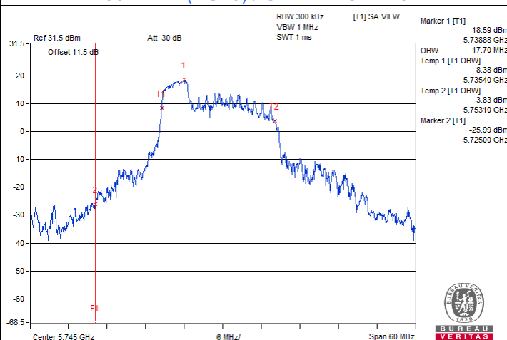
802.11ax (RU52) / Chain 1 : CH 149
