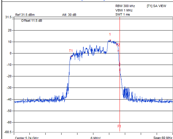
802.11ax (RU52) / Chain 0 : CH 48
