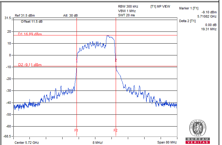
802.11ax (RU52) : CH 144 (U-NII-2C)
