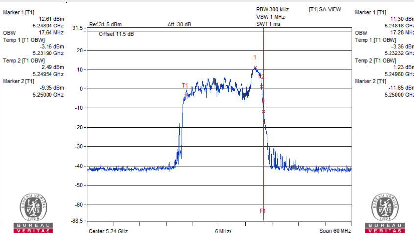
802.11ax (RU26) / Chain 1 : CH 48
