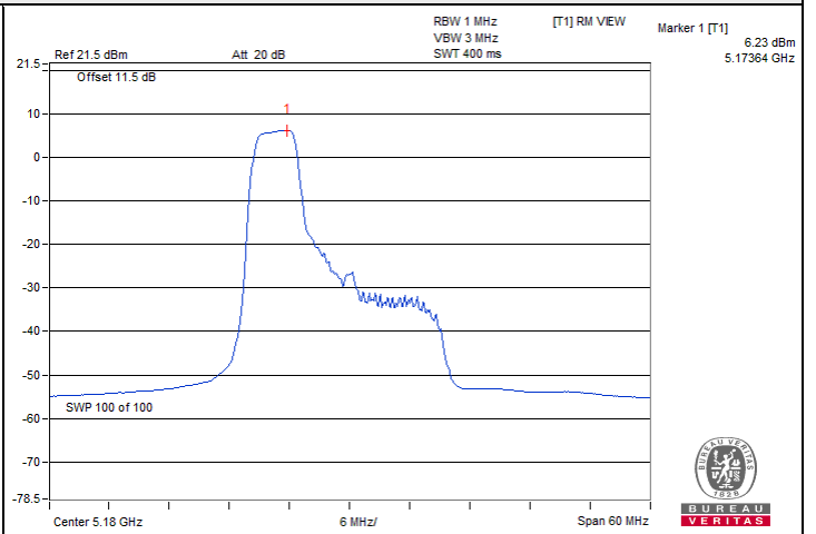
802.11ax (RU52) / Chain0 : CH 36
