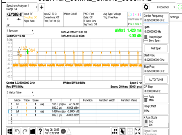
802.11ax_160MHz_Chain0_6025MHz
