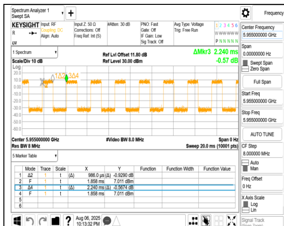
802.11ax 20MHz Chain0 5955MHz
