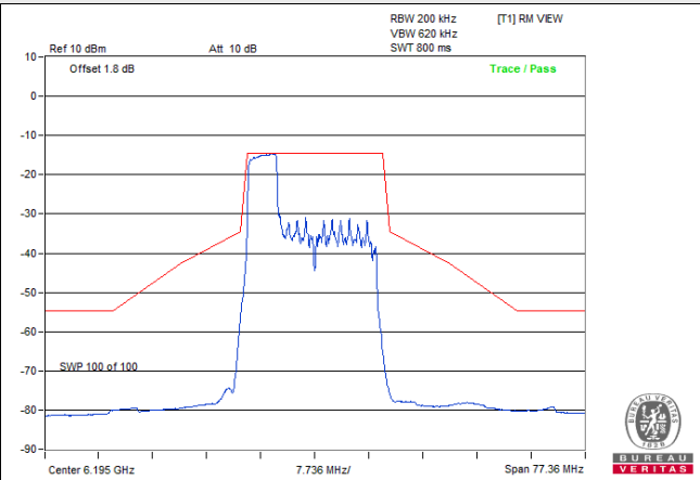
802.11be (EHT20) 52-tone RU / Chain 0: CH 49
