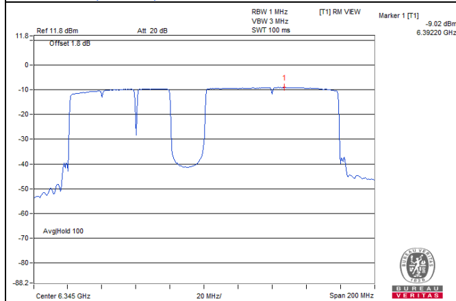
802.11be (EHT160) 996+484+242-tone MRU / Chain 0: CH 79
