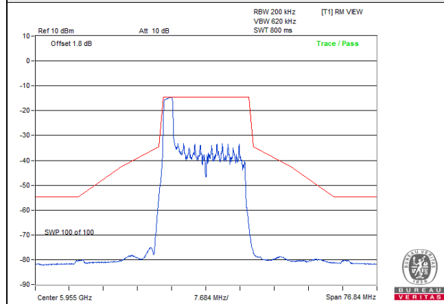
802.11be (EHT20) 26-tone RU / Chain 0: CH 1
