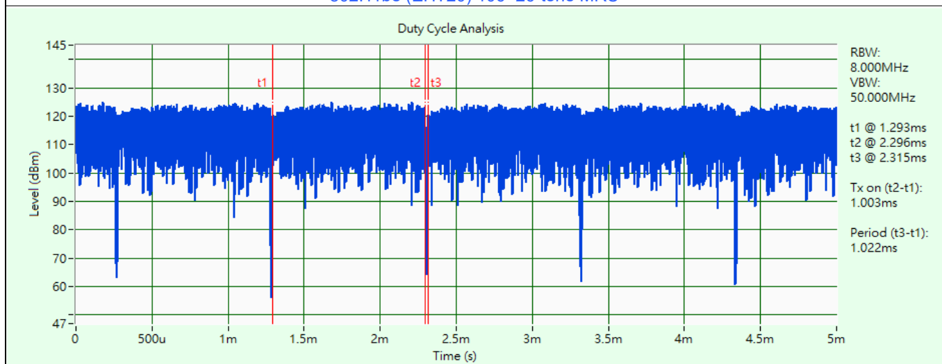
802.11be (EHT80) 484+242-tone MRU
