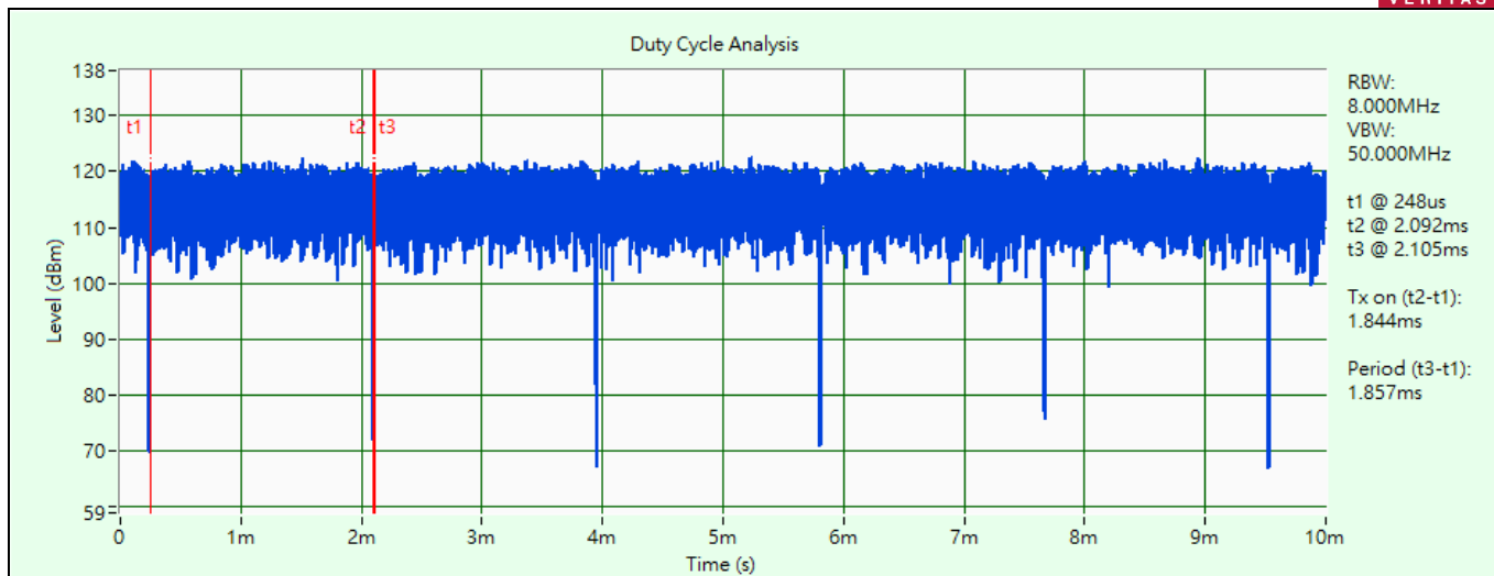
802.11be (EHT160) 996+484-tone MRU
