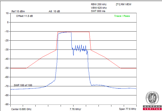
802.11be (EHT20) 106-tone RU: CH 149
