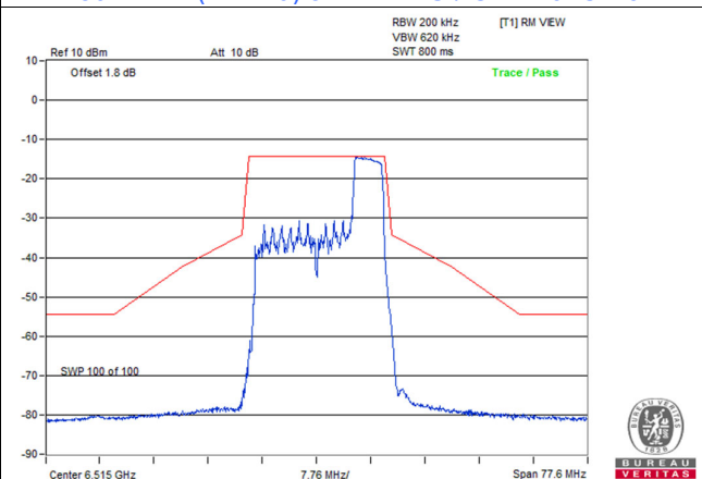
802.11be (EHT20) 52-tone RU / Chain 0: CH 113
