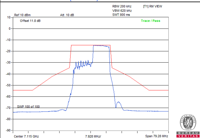
802.11be (EHT20) 106-tone RU: CH 233
