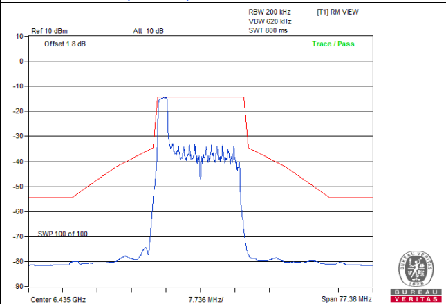
802.11be (EHT20) 26-tone RU / Chain 0: CH 97
