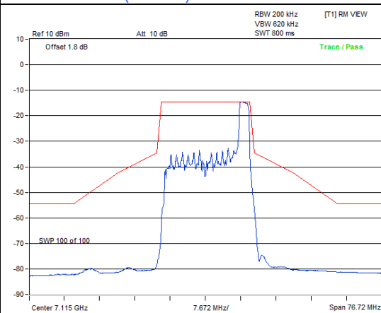
802.11be (EHT20) 26-tone RU / Chain 1: CH 233
