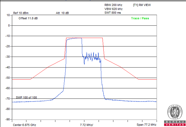
802.11be (EHT20) 106-tone RU: CH 185
