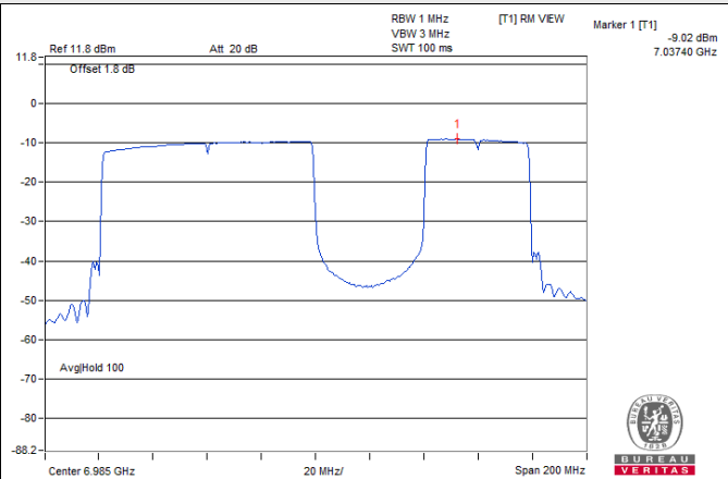
802.11be (EHT160) 996+484-tone MRU / Chain 0: CH 207
