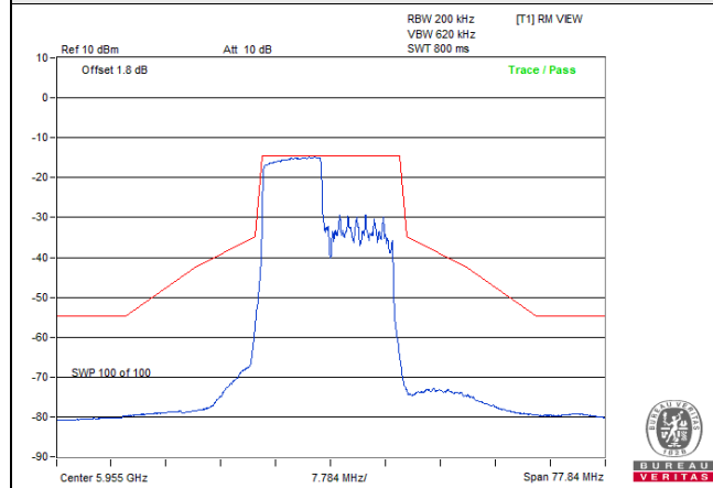
802.11be (EHT20) 106-tone RU / Chain 0: CH 1
