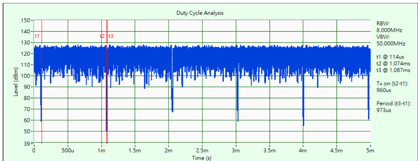
802.11a
