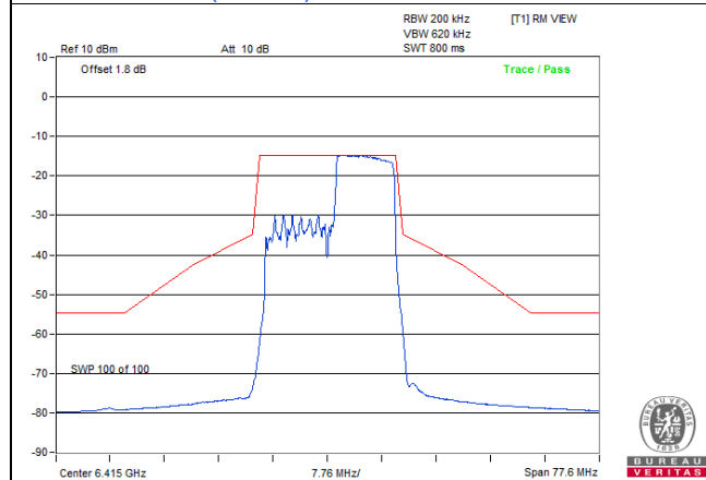
802.11be (EHT20) 106-tone RU / Chain 0: CH 93
