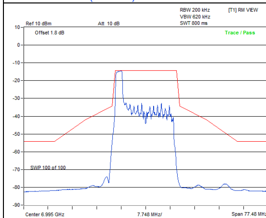
802.11be (EHT20) 26-tone RU / Chain 1: CH 209
