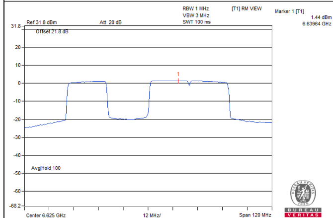
802.11be (EHT80) 484+242-tone MRU / Chain 1: CH 135
