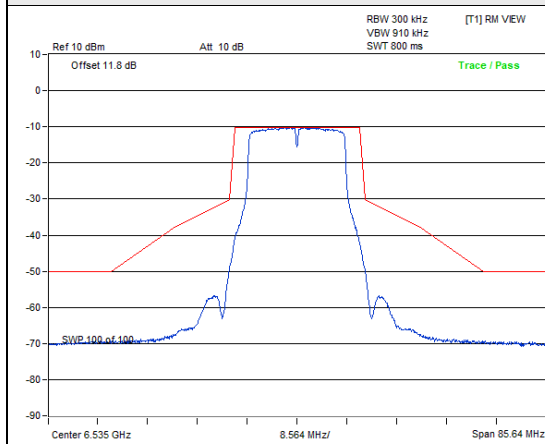
802.11a: CH 117
