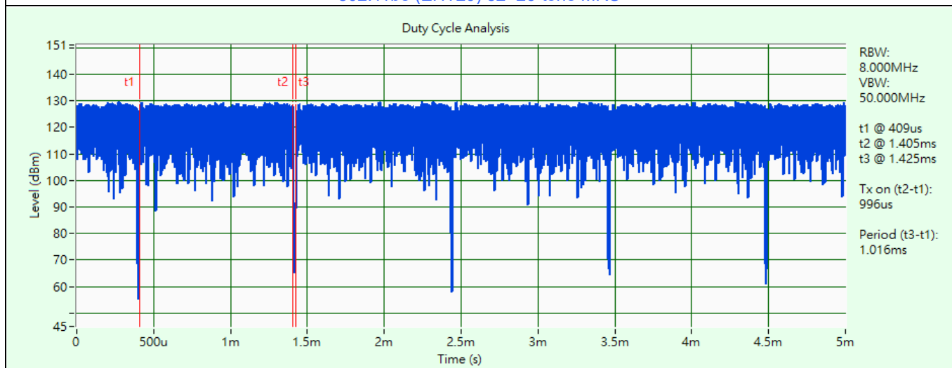
802.11be (EHT20) 106+26-tone MRU
