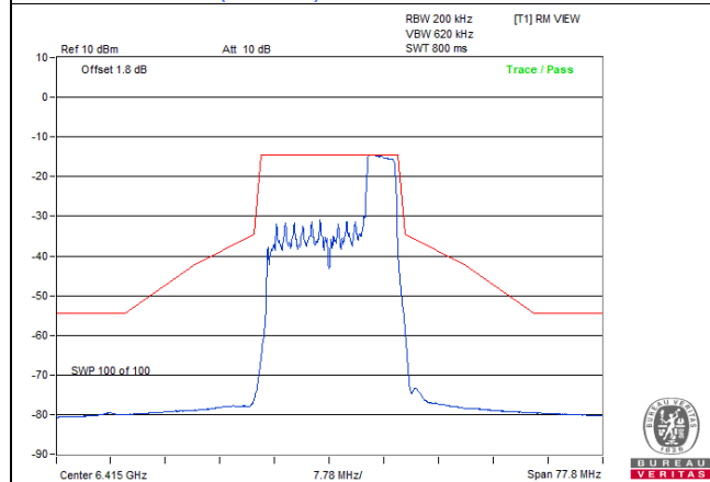
802.11be (EHT20) 52-tone RU / Chain 0: CH 93
