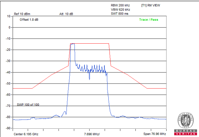
802.11be (EHT20) 26-tone RU / Chain 0: CH 49
