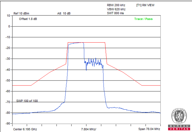
802.11be (EHT20) 106-tone RU / Chain 0: CH 49
