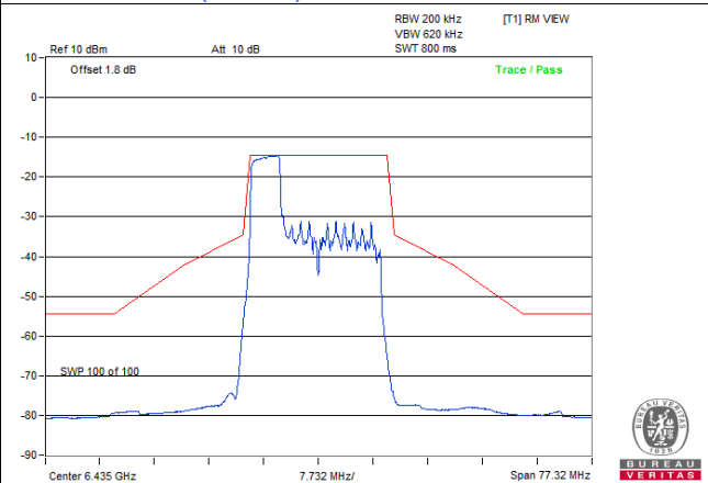
802.11be (EHT20) 52-tone RU / Chain 0: CH 97
