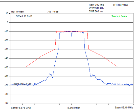
802.11a: CH 185
