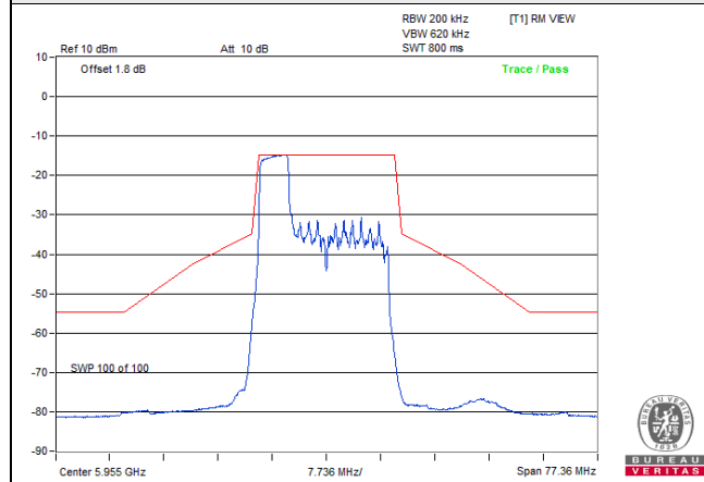
802.11be (EHT20) 52-tone RU / Chain 0: CH 1
