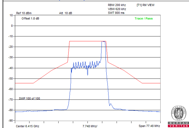
802.11be (EHT20) 26-tone RU / Chain 0: CH 93
