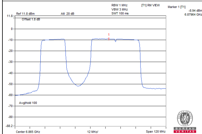
802.11be (EHT80) 484+242-tone MRU / Chain 0: CH 183
