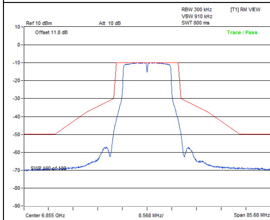
802.11a: CH 181
