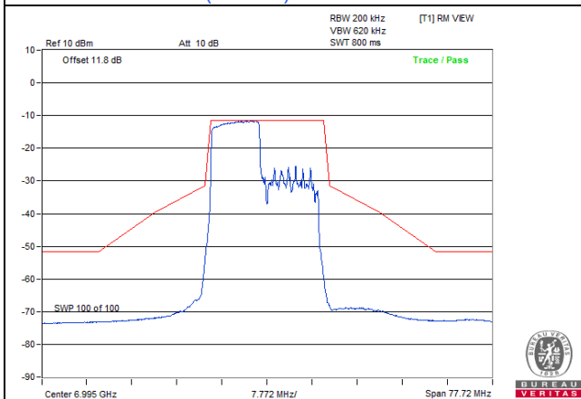
802.11be (EHT20) 106-tone RU: CH 209
