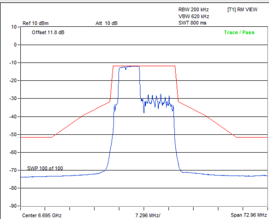
802.11be (EHT20) 52+26-tone MRU: CH 149
