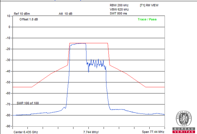
802.11be (EHT20) 106-tone RU / Chain 0: CH 97
