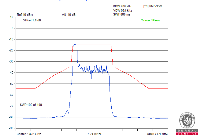
802.11be (EHT20) 26-tone RU / Chain 0: CH 105
