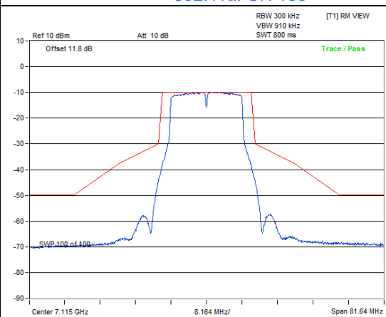
802.11a: CH 233
