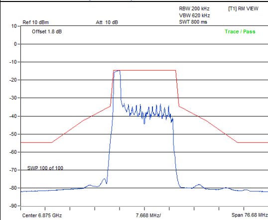
802.11be (EHT20) 26-tone RU / Chain 1: CH 185
