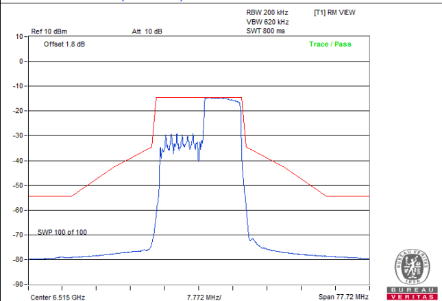
802.11be (EHT20) 106-tone RU / Chain 0: CH 113
