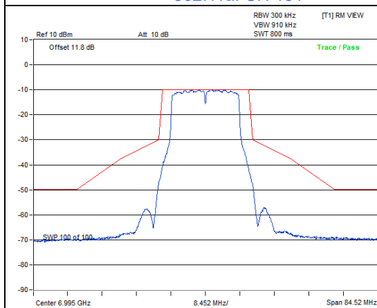
802.11a: CH 209
