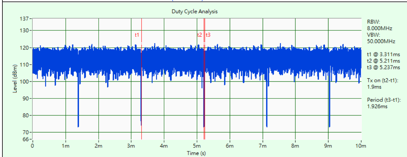
802.11be (EHT160) 996+484+242-tone MRU
