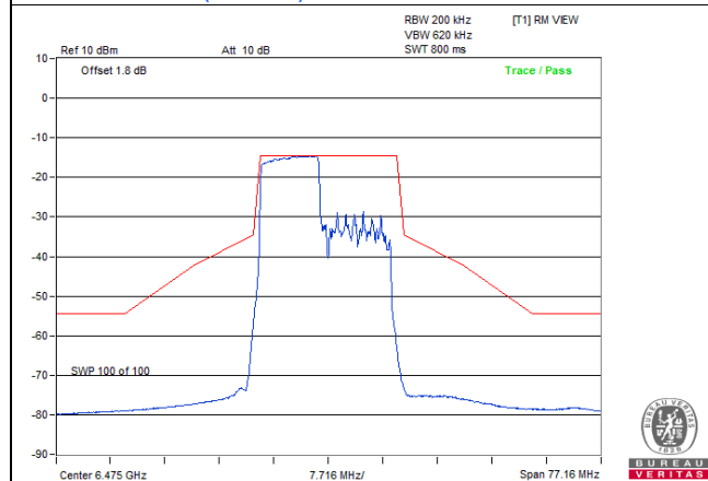
802.11be (EHT20) 106-tone RU / Chain 0: CH 105
