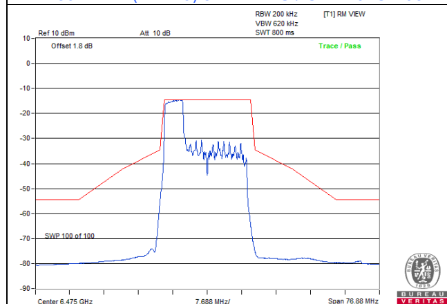
802.11be (EHT20) 52-tone RU / Chain 0: CH 105
