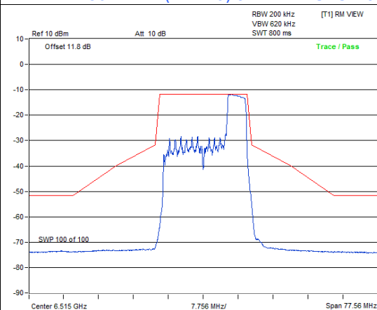
802.11be (EHT20) 52-tone RU: CH 113
