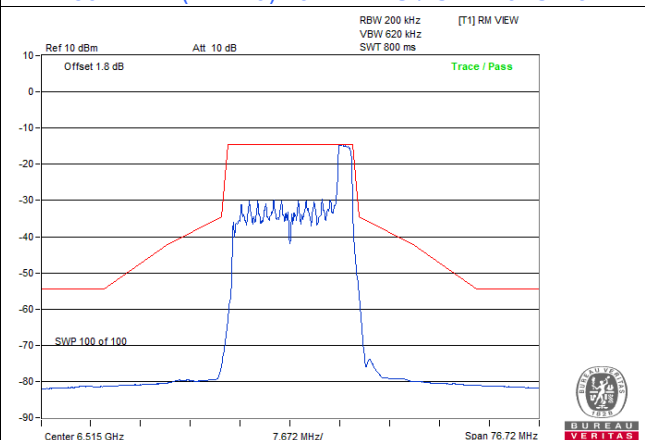
802.11be (EHT20) 26-tone RU / Chain 0: CH 113
