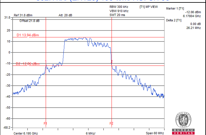
802.11be (EHT20) 106+26-tone MRU: CH 49
