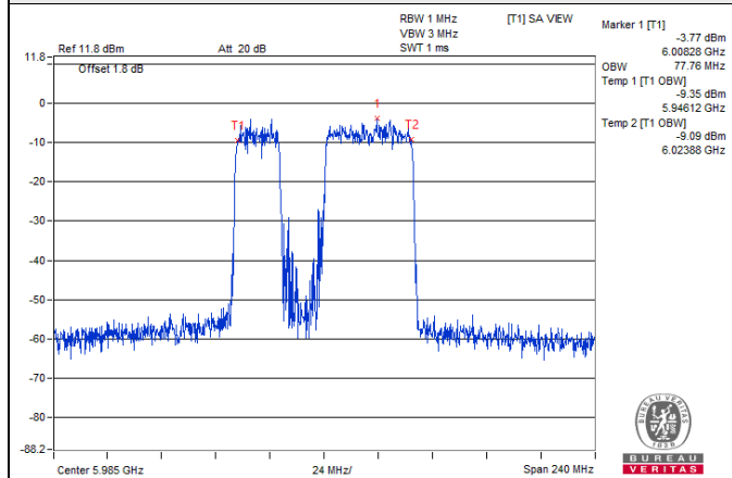
802.11be (EHT80) 484+242-tone MRU / Chain 1: CH 7
