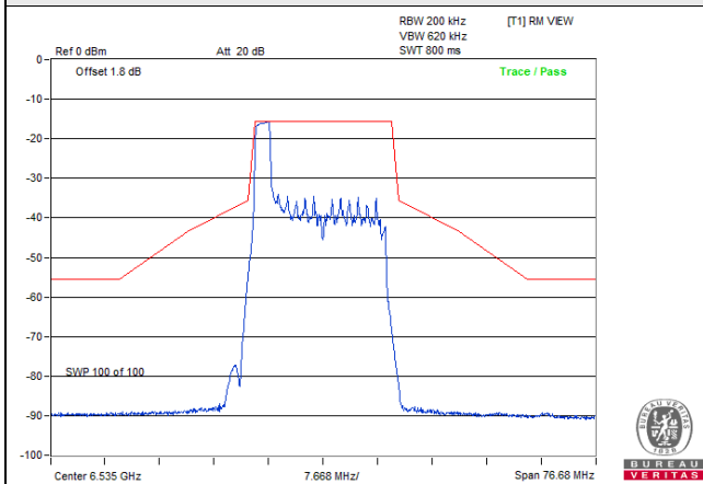
802.11be (EHT20) 26-tone RU: CH 117
