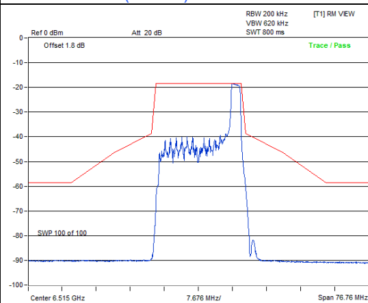
802.11be (EHT20) 26-tone RU / Chain 1: CH 113
