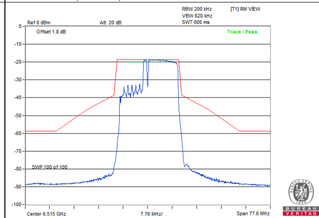
802.11be (EHT20) 106+26-tone MRU / Chain 0: CH 113
