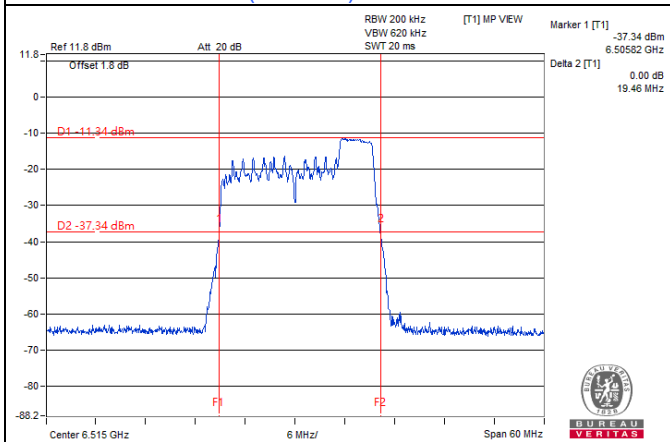
802.11be (EHT20) 52-tone RU / Chain 1: CH 113
