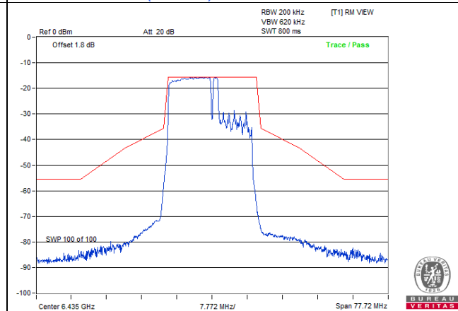
802.11be (EHT20) 106+26-tone MRU: CH 97
