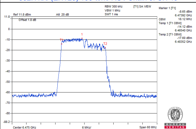
802.11be (EHT20) 106+26-tone MRU / Chain 0: CH 105
