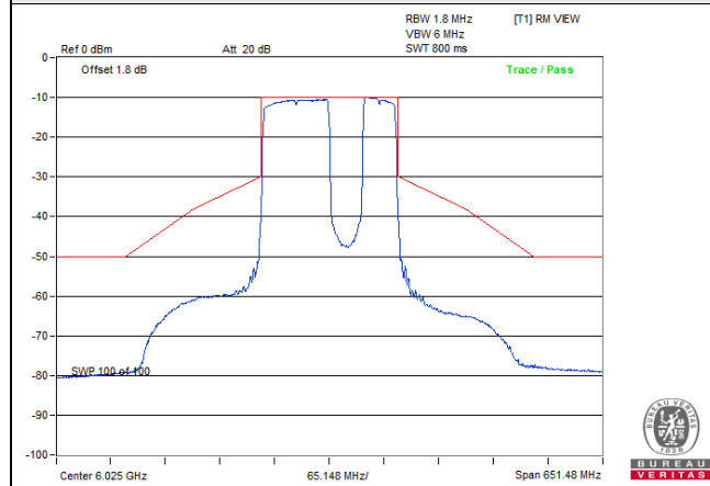
802.11be (EHT160) 996+484-tone MRU: CH 15
