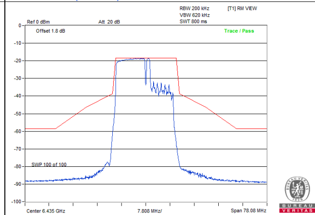
802.11be (EHT20) 106+26-tone MRU / Chain 0: CH 97
