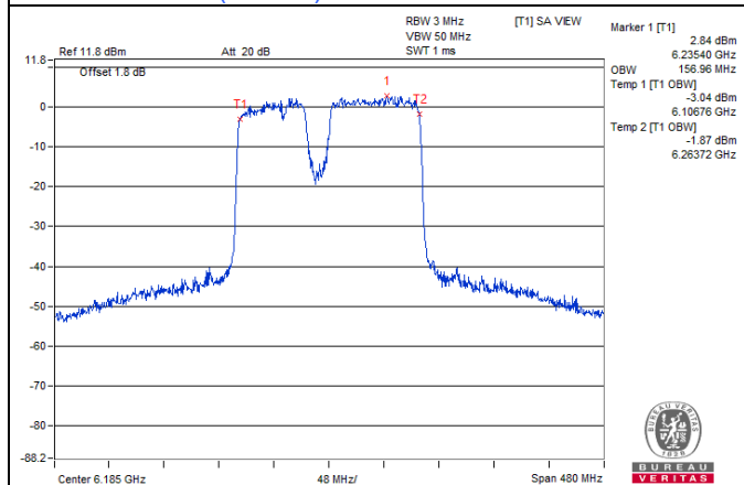
802.11be (EHT160) 996+484+242-tone MRU: CH 47
