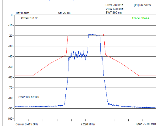
802.11be (EHT20) 52+26-tone MRU / Chain 0: CH 93
