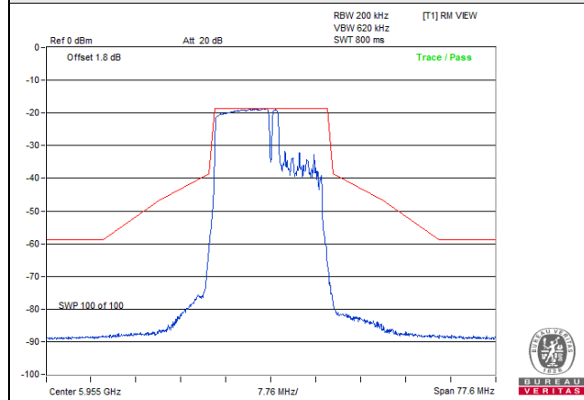
802.11be (EHT20) 106+26-tone MRU / Chain 0: CH 1
