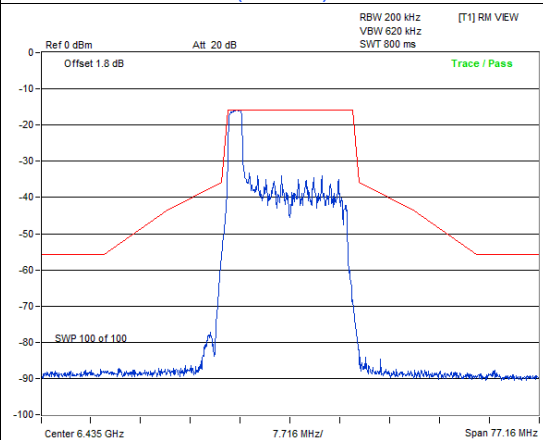
802.11be (EHT20) 26-tone RU: CH 97
