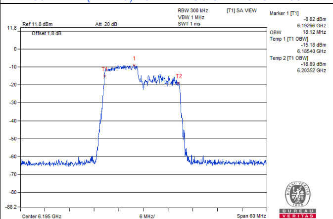
802.11be (EHT20) 106-tone RU / Chain 0: CH 49
