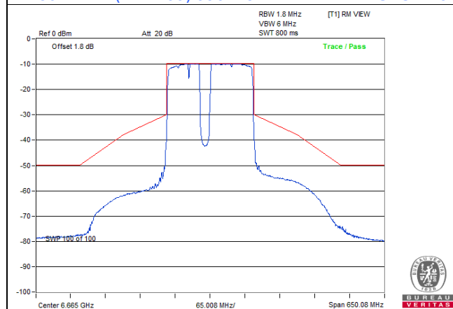
802.11be (EHT160) 996+484+242-tone MRU: CH 143
