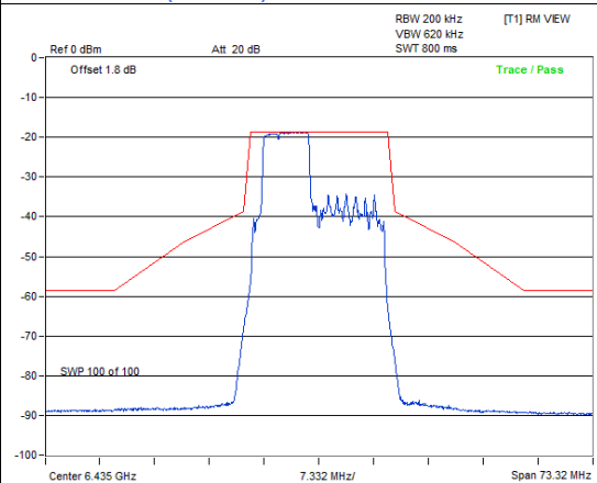
802.11be (EHT20) 52+26-tone MRU / Chain 0: CH 97
