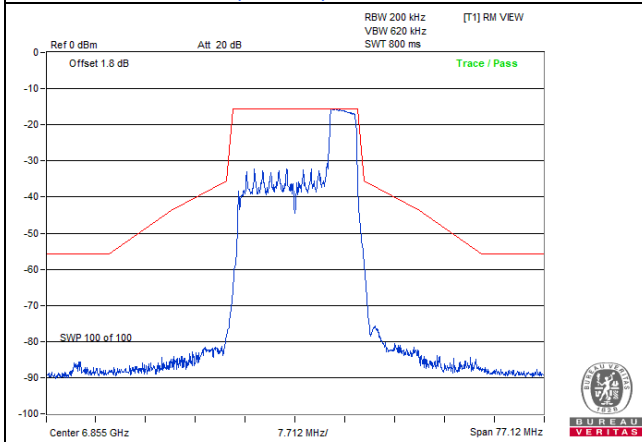
802.11be (EHT20) 52-tone RU: CH 181
