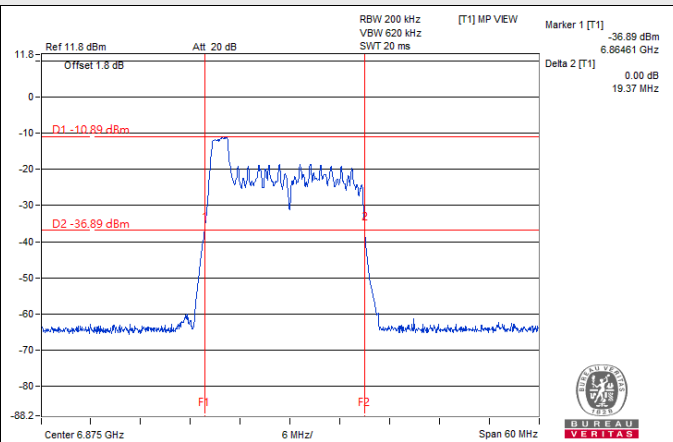
802.11be (EHT20) 26-tone RU / Chain 1: CH 185
