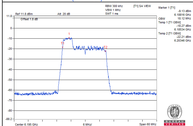
802.11be (EHT20) 52-tone RU / Chain 0: CH 49
