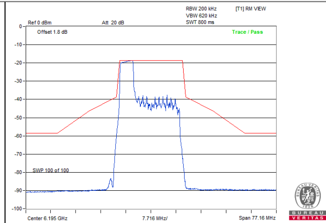
802.11be (EHT20) 52-tone RU / Chain 0: CH 49
