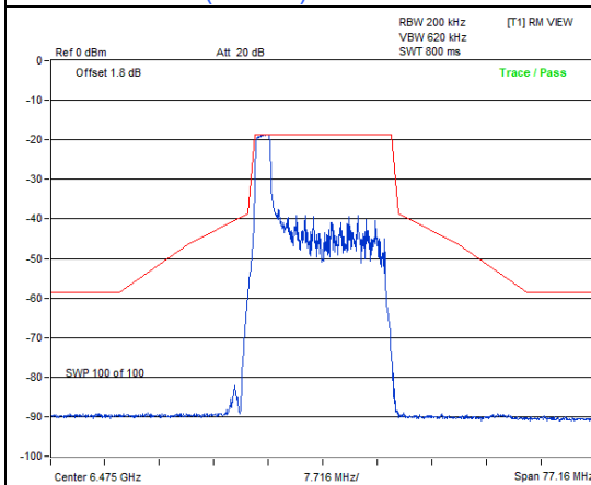
802.11be (EHT20) 26-tone RU / Chain 1: CH 105
