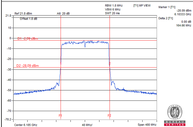
802.11be (EHT160) / Chain 1: CH 47
