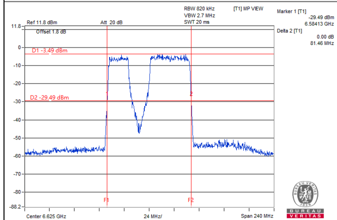
802.11be (EHT80) 484+242-tone MRU / Chain 0: CH 135
