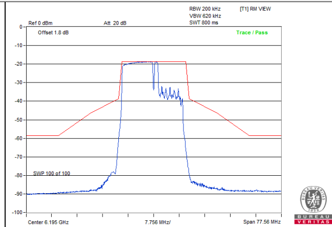
802.11be (EHT20) 106+26-tone MRU / Chain 0: CH 49
