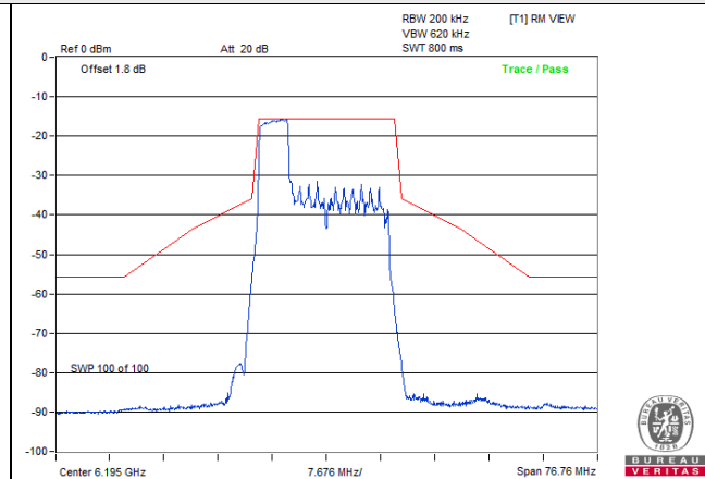
802.11be (EHT20) 52-tone RU: CH 49
