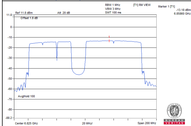
802.11be (EHT160) 996+484+242-tone MRU: CH 175
