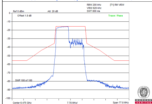
802.11be (EHT20) 106-tone RU: CH 105
