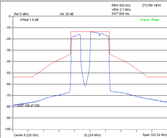
802.11be (EHT80) 484+242-tone MRU / Chain 0: CH 55
