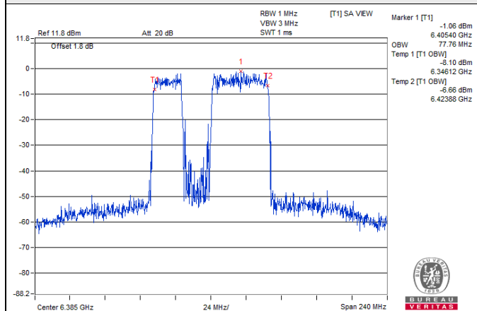
802.11be (EHT80) 484+242-tone MRU: CH 87
