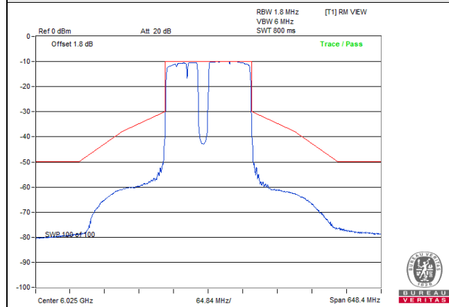
802.11be (EHT160) 996+484+242-tone MRU: CH 15
