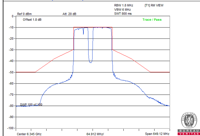
802.11be (EHT160) 996+484+242-tone MRU: CH 79
