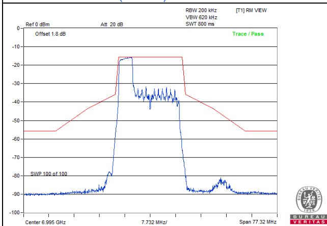
802.11be (EHT20) 52-tone RU: CH 209
