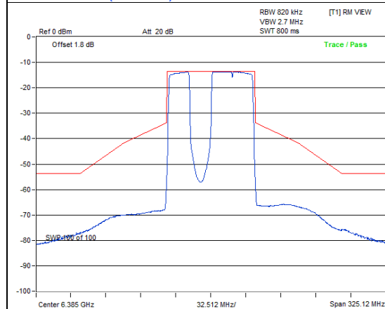
802.11be (EHT80) 484+242-tone MRU / Chain 0: CH 87
