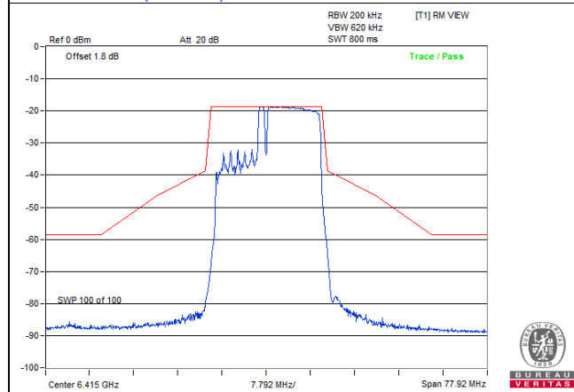
802.11be (EHT20) 106+26-tone MRU / Chain 0: CH 93
