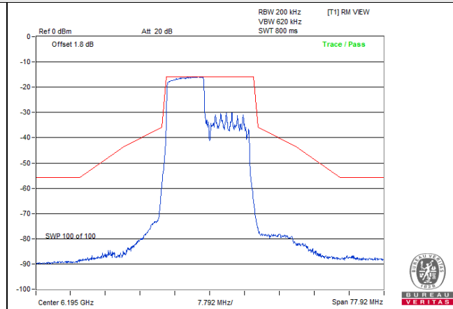
802.11be (EHT20) 106-tone RU: CH 49
