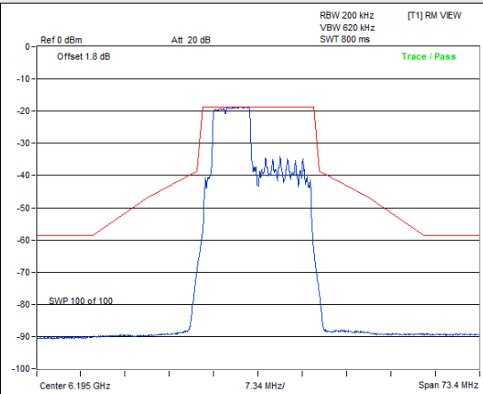
802.11be (EHT20) 52+26-tone MRU / Chain 0: CH 49
