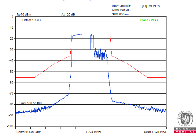
802.11be (EHT20) 106+26-tone MRU: CH 105
