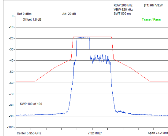
802.11be (EHT20) 52+26-tone MRU / Chain 0: CH 1
