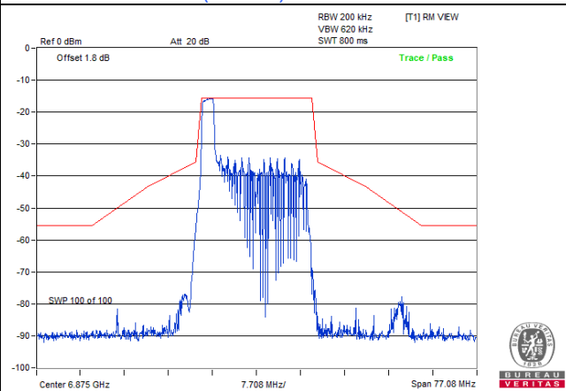
802.11be (EHT20) 26-tone RU: CH 185
