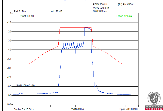
802.11be (EHT20) 52-tone RU: CH 93
