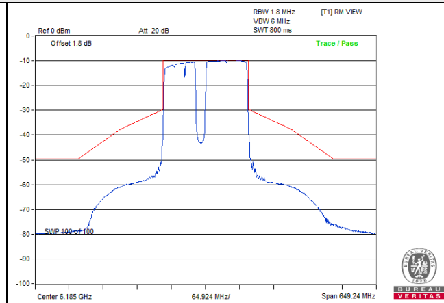
802.11be (EHT160) 996+484+242-tone MRU: CH 47
