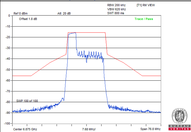
802.11be (EHT20) 52-tone RU: CH 185
