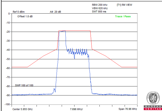
802.11be (EHT20) 52-tone RU / Chain 1: CH 1
