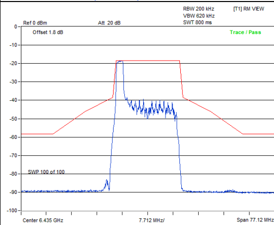
802.11be (EHT20) 26-tone RU / Chain 1: CH 97
