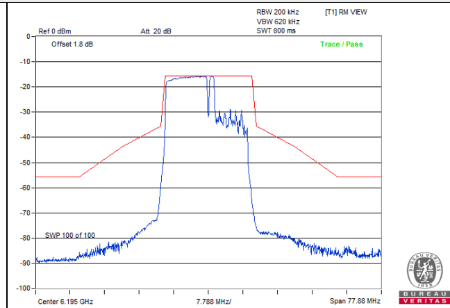
802.11be (EHT20) 106+26-tone MRU: CH 49
