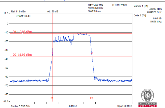
802.11be (EHT20) 106-tone RU / Chain 1: CH 181
