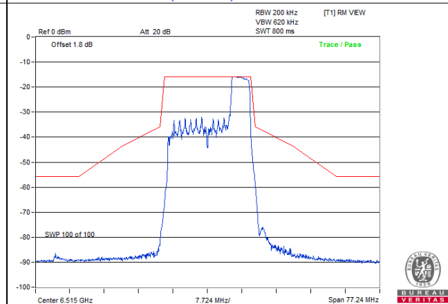
802.11be (EHT20) 52-tone RU: CH 113
