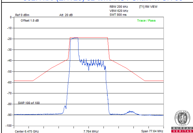
802.11be (EHT20) 52-tone RU / Chain 1: CH 105
