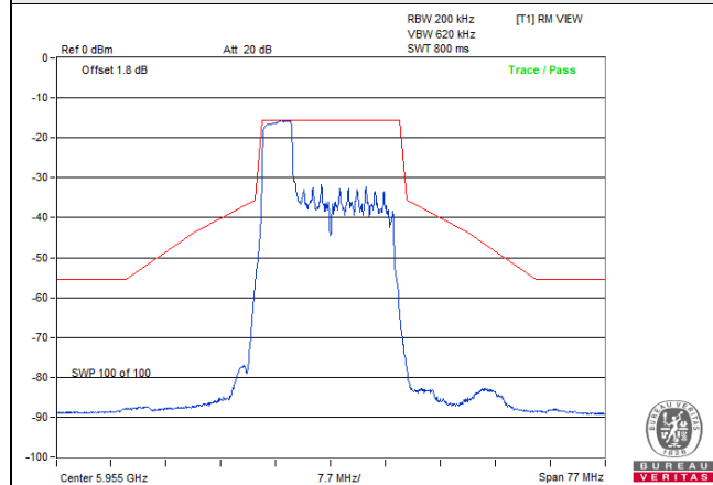
802.11be (EHT20) 52-tone RU: CH 1
