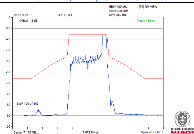
802.11be (EHT20) 26-tone RU: CH 233
