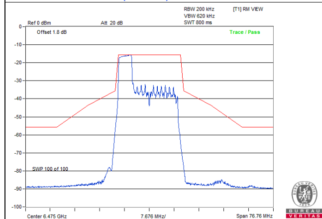
802.11be (EHT20) 52-tone RU: CH 105
