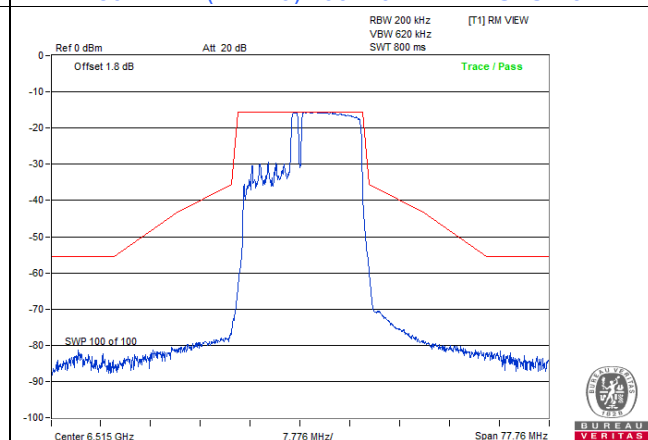
802.11be (EHT20) 106+26-tone MRU: CH 113
