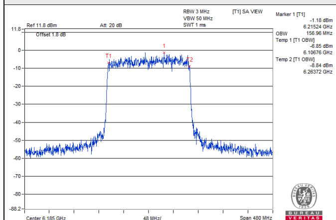
802.11be (EHT160) / Chain 1: CH 47
