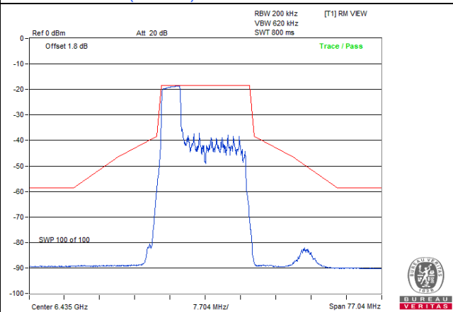
802.11be (EHT20) 52-tone RU / Chain 1: CH 97
