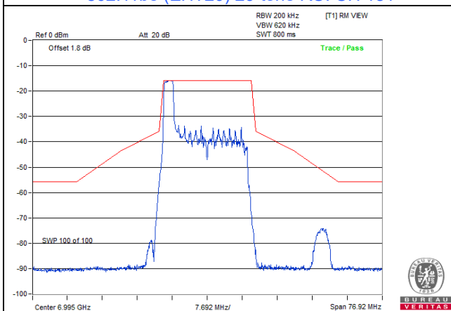
802.11be (EHT20) 26-tone RU: CH 209
