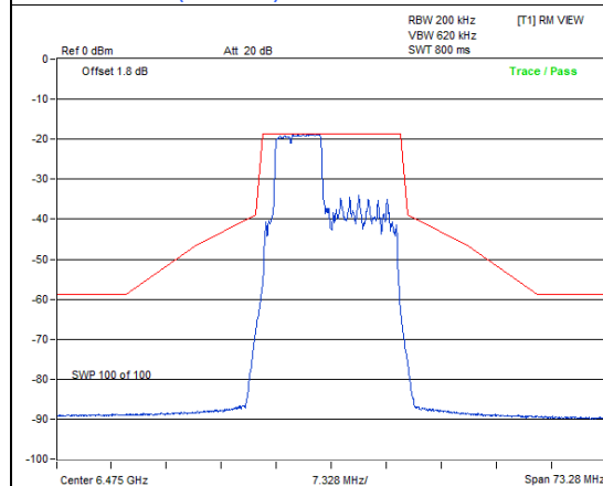
802.11be (EHT20) 52+26-tone MRU / Chain 0: CH 105
