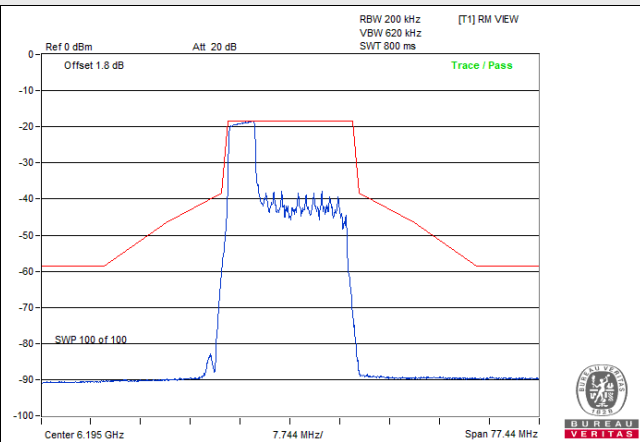
802.11be (EHT20) 52-tone RU / Chain 1: CH 49
