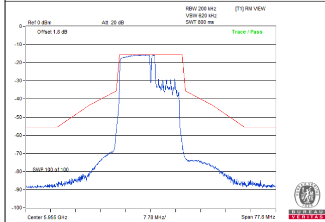
802.11be (EHT20) 106+26-tone MRU: CH 1
