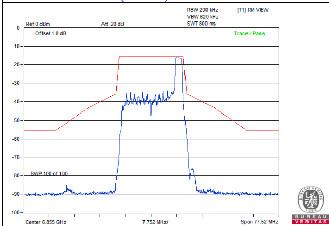
802.11be (EHT20) 26-tone RU: CH 181
