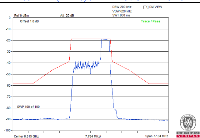
802.11be (EHT20) 52-tone RU / Chain 1: CH 113
