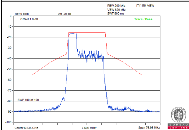
802.11be (EHT20) 52-tone RU: CH 117
