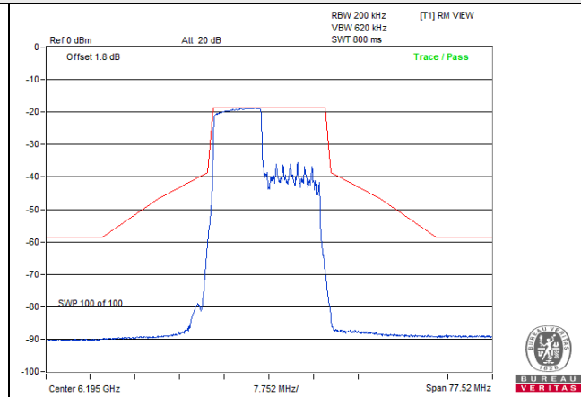
802.11be (EHT20) 106-tone RU / Chain 0: CH 49
