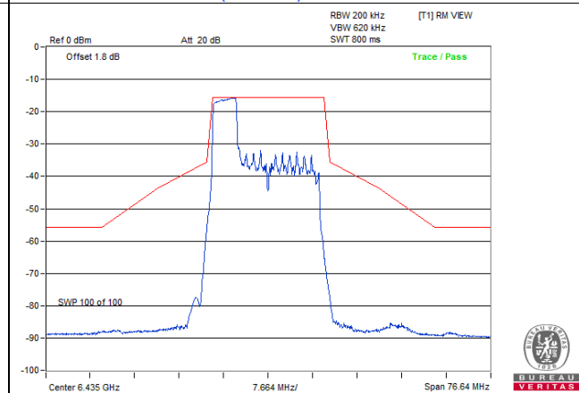
802.11be (EHT20) 52-tone RU: CH 97
