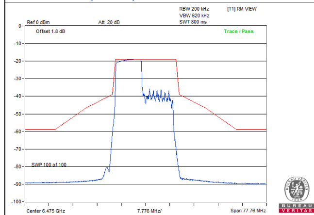
802.11be (EHT20) 106-tone RU / Chain 0: CH 105
