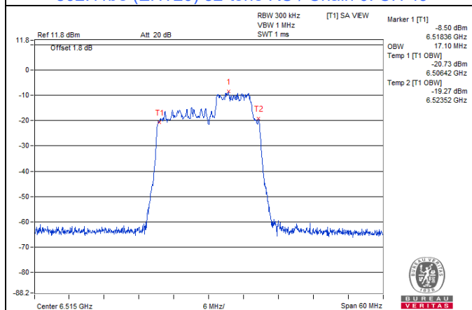
802.11be (EHT20) 52+26-tone MRU / Chain 0: CH 113
