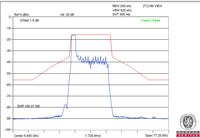
802.11be (EHT20) 26-tone RU: CH 149
