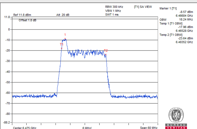
802.11be (EHT20) 26-tone RU / Chain 0: CH 105
