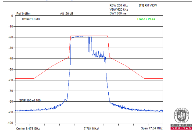
802.11be (EHT20) 106+26-tone MRU / Chain 0: CH 105
