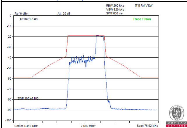
802.11be (EHT20) 52-tone RU / Chain 1: CH 93
