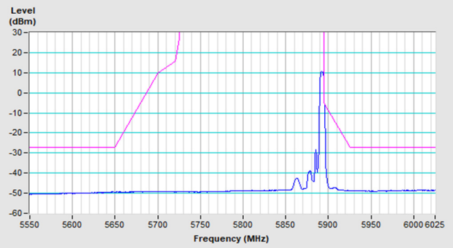
Vertical (Average)
