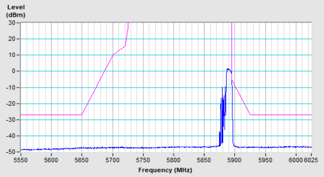
Horizontal (Average)
