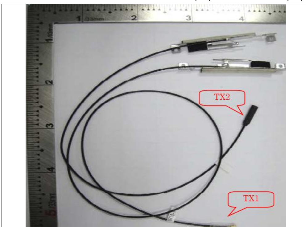
Antenna 3: Brand: WGT / Model: SKA91WMPB02+A (Tx1) & SKA91WMPB01+A (Tx2)
