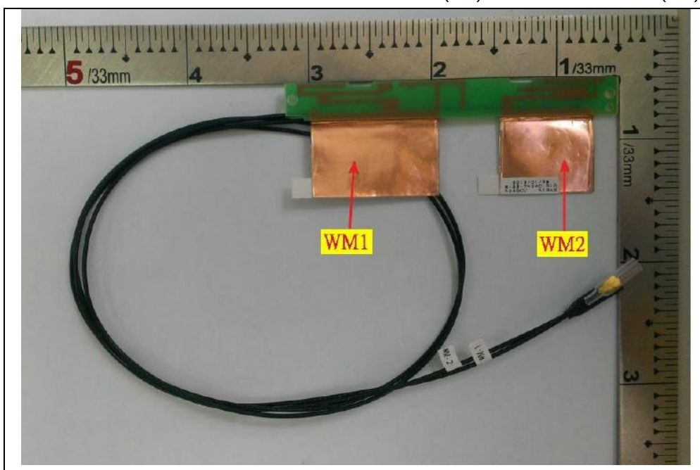
Antenna 8: Brand: WGT / Model: SKW2UWMPB01+A (Tx1) & SKW2UWMPB01+A (Tx2)
