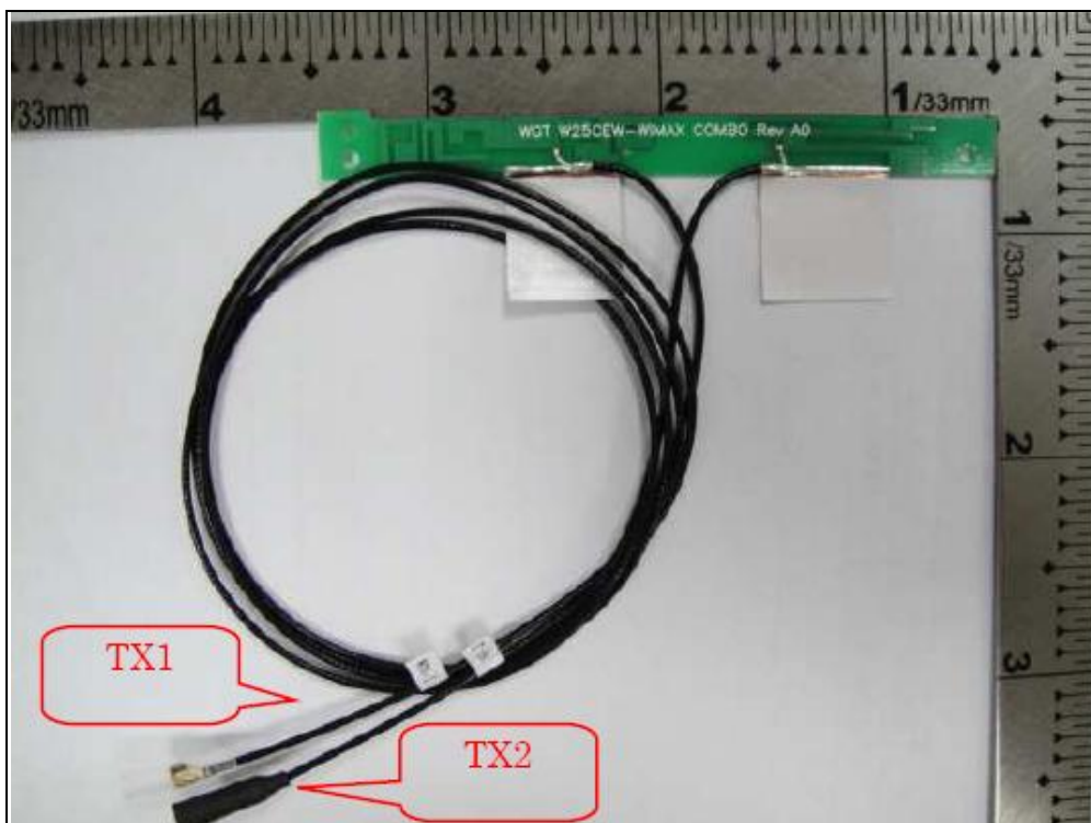
Antenna 9: Brand: WGT / Model: SKW25WMPB01+A (Tx1) & SKW25WMPB01+A (Tx2)
