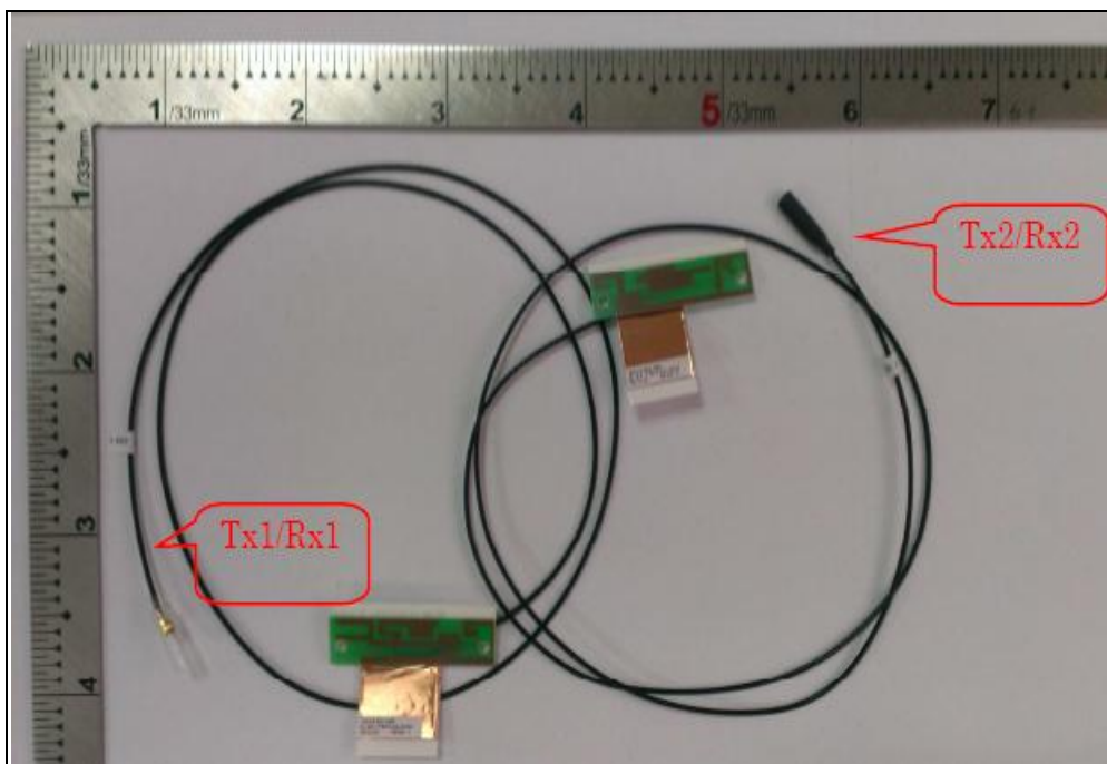
Antenna 21: Brand: WGT / Model: SKW10WMPB01+A (Tx1) & SKW10WMPB02+A (Tx2)
