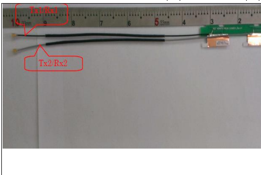
Antenna 33: Brand: WGT / Model: SK94TWMPB01+D (TX1) & SK94TWMPB01+D (TX2)
