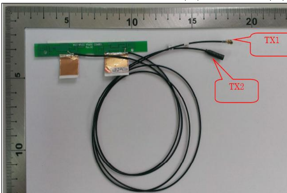
Antenna 26: Brand: WGT / Model: SK65EWMPB01+A (Tx1) & SK650WMPB02+A (Tx2)
