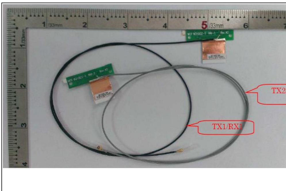
Antenna 22: Brand: WGT / Model: SKCZTWMPB01+A (Tx1) & SKCZTWMPB02+A (Tx2)
