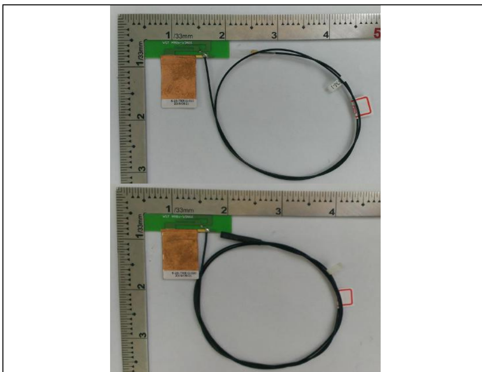
Antenna 7: Brand: WGT / Model: SK81WMPB01+A (Tx1) & SK81WMPB02+A (Tx2)
