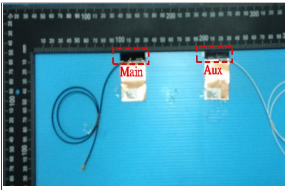
Antenna 41: Brand: INPAQ / Model: WA-P-LB-02-121 (Main) & WA-P-LB-01-071 (Aux)
