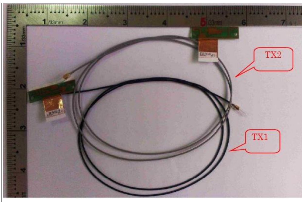
Antenna 17: Brand: WGT / Model: SKW23WMPB01+A (Tx1) & SKW23WMPB02+A (Tx2)
