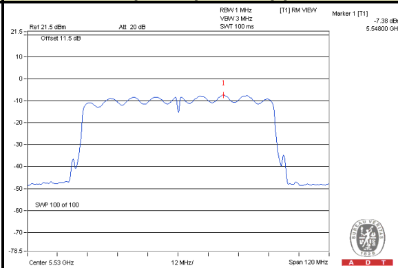
802.11ac (VHT80) / Chain(0) : CH106
