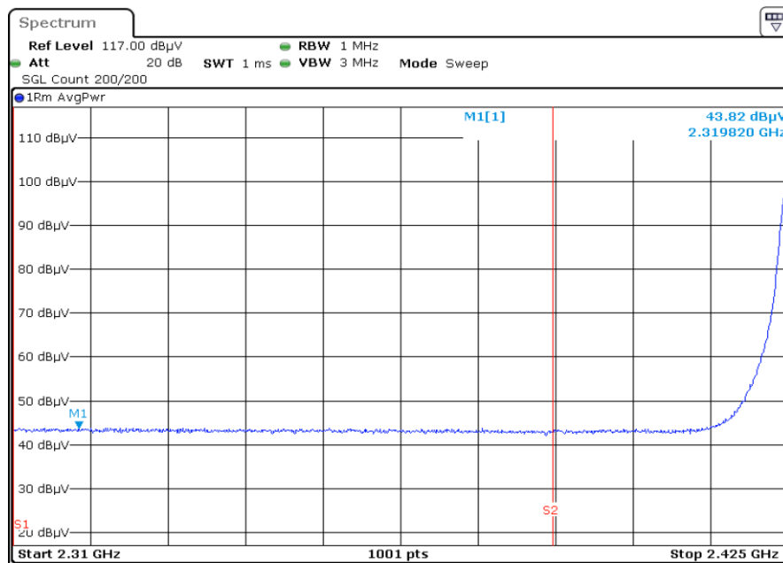
2425.0 F1 RestrictedBand Vertical AVG
