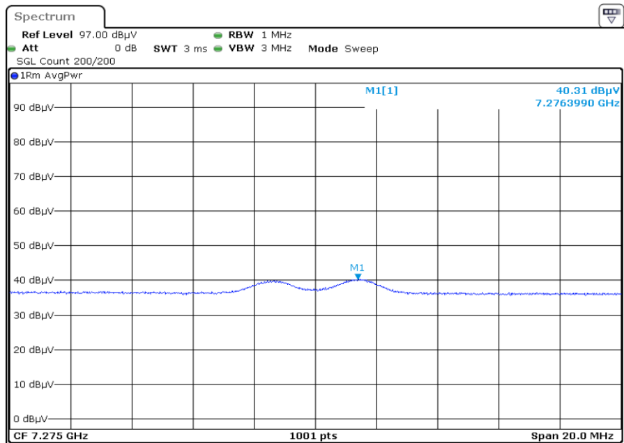
F1 X3 7275.0 Harmonic Horizontal AVG
