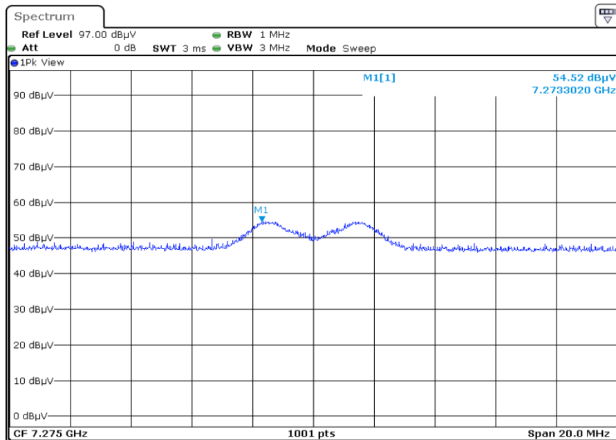
F1 X3 7275.0 Harmonic Vertical PEAK
