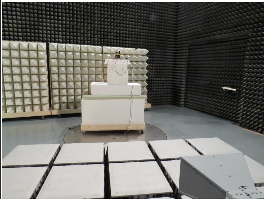
VIEW A4
