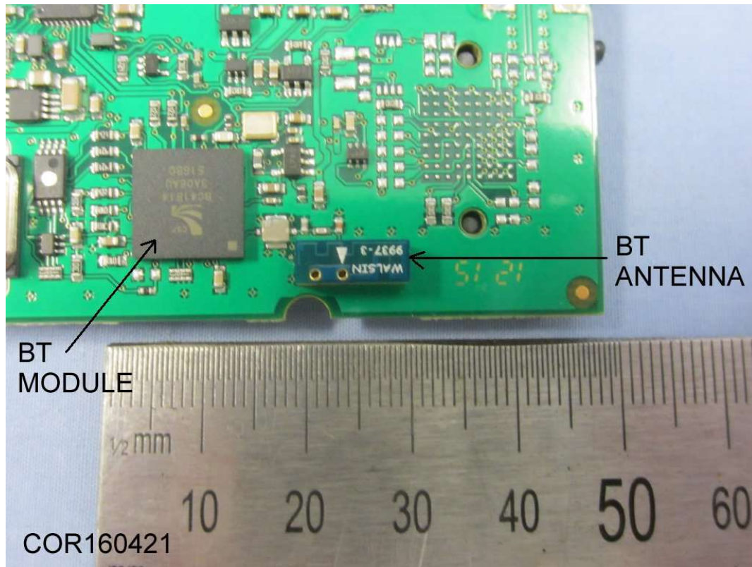
BT Module & Antenna
