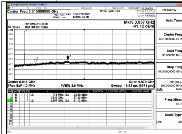
Band13 5MHz QPSK RB1 0 CH23205 below 18G
