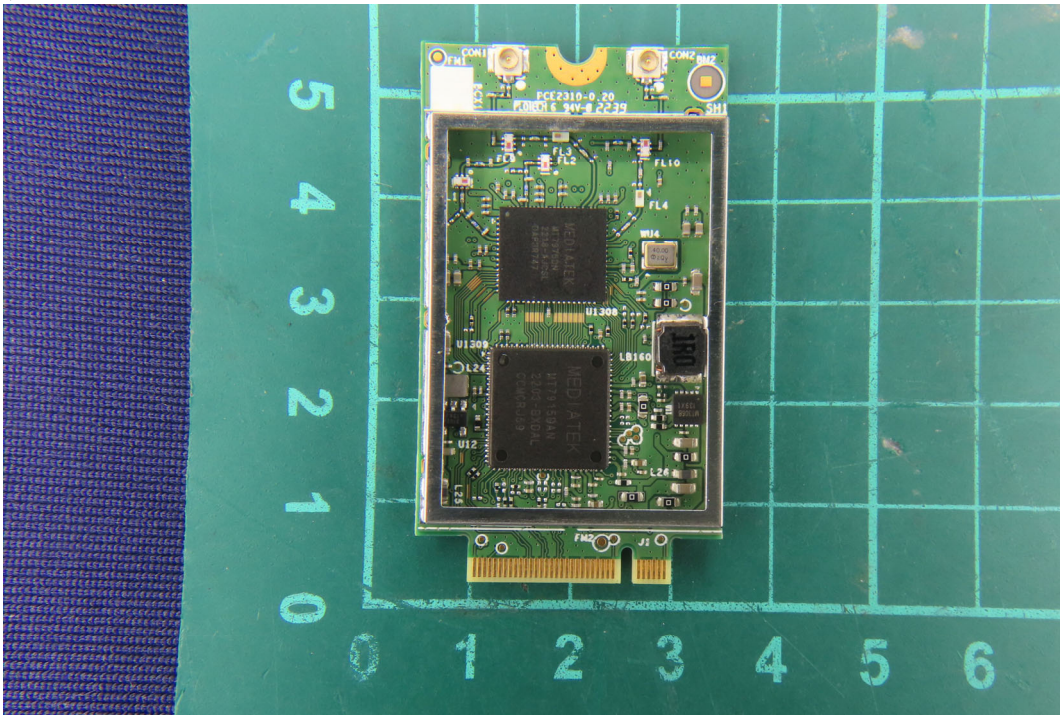
(2) EUT Photo
