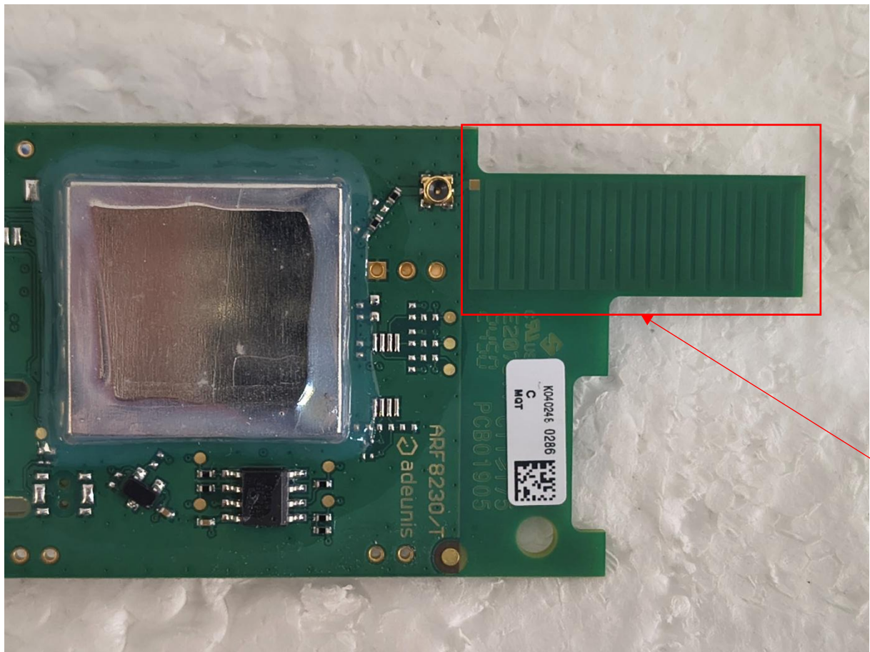
Module alone
