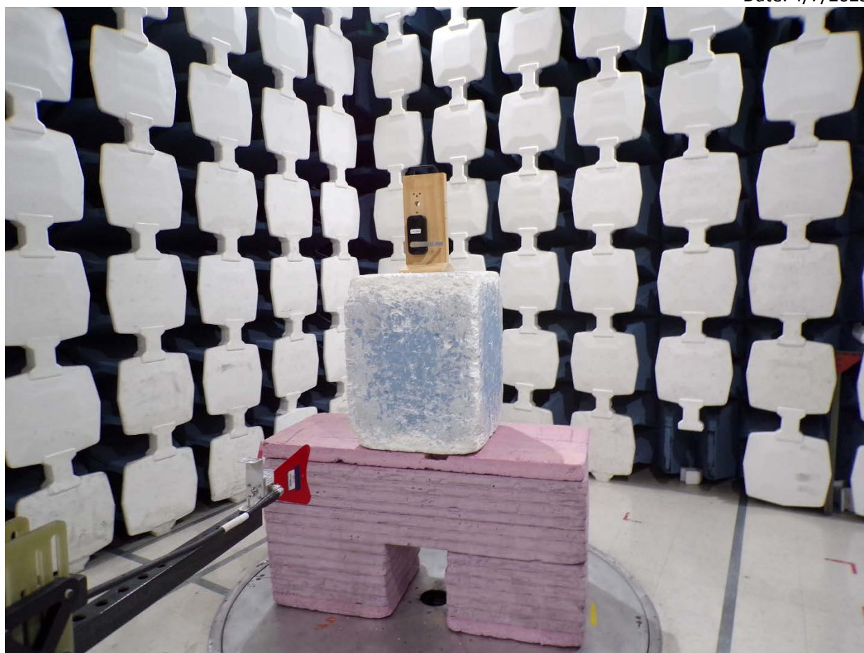
6-18GHz
