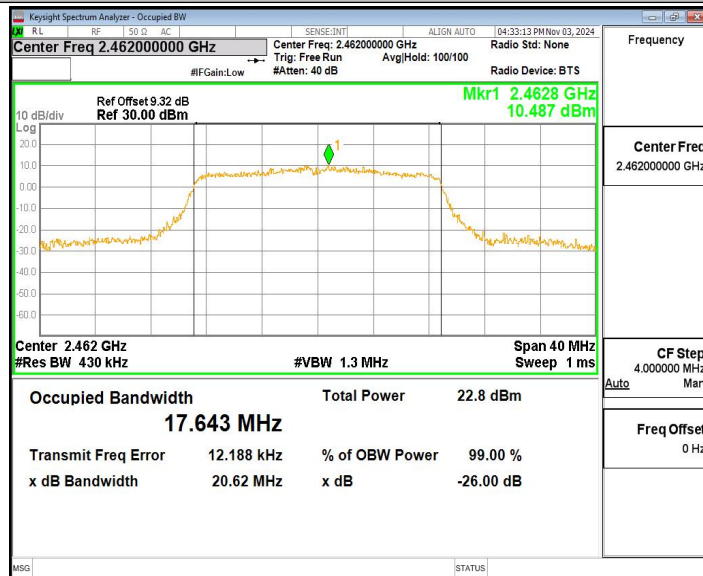
11N20MIMO_Ant9_2462
