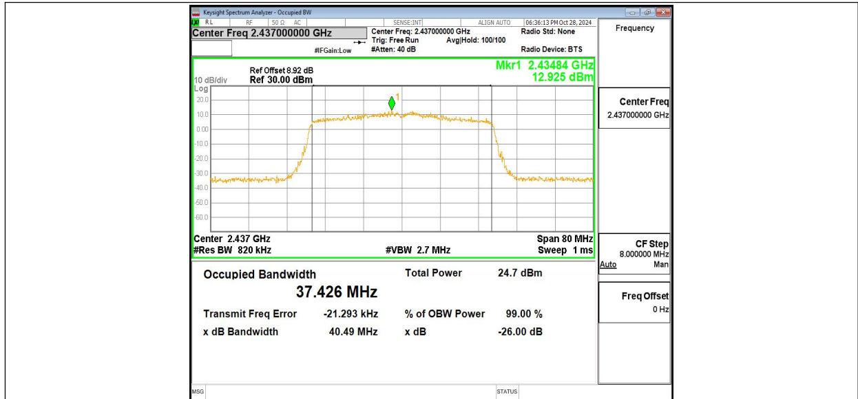
11AX40MIMO_Ant9_2437
