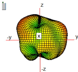
WIFI 6E ( 6200 MHz)
