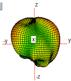
WIFI 5G ( 5600 MHz)
