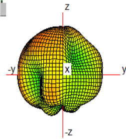
WIFI 6E ( 6200 MHz)
