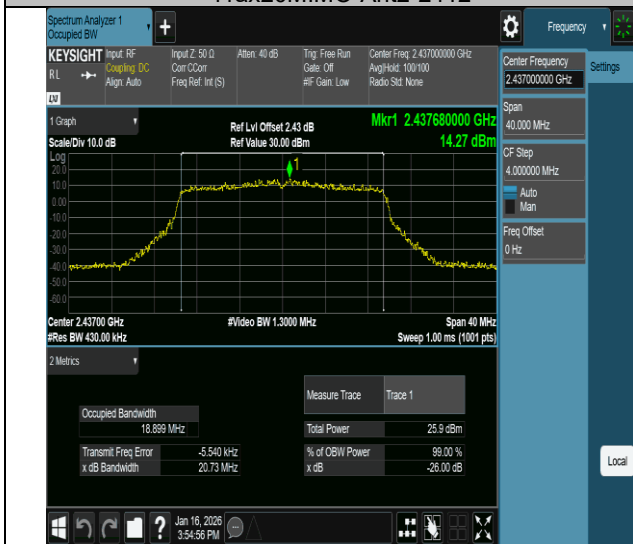
11ax20MIMO-Ant2-2437
