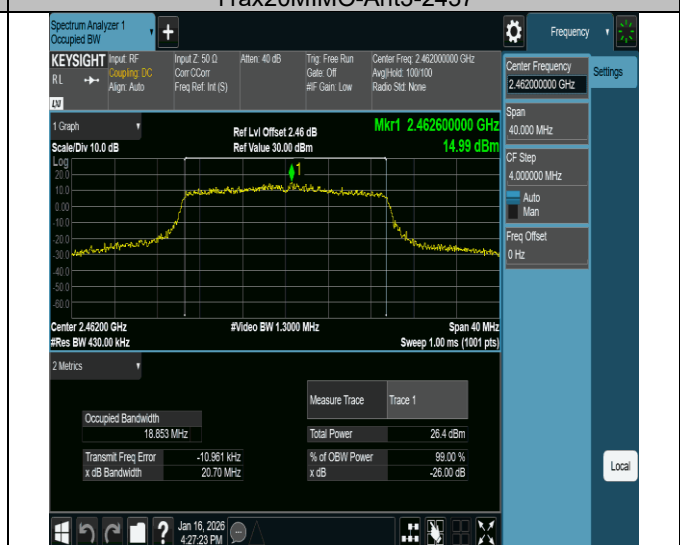
11ax20MIMO-Ant3-2462
