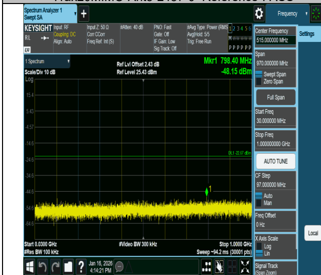
11ax20MIMO-Ant3-2437-30~1000-PASS
