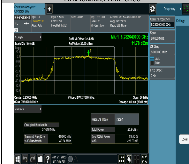
11ax40MIMO-Ant2-5230
