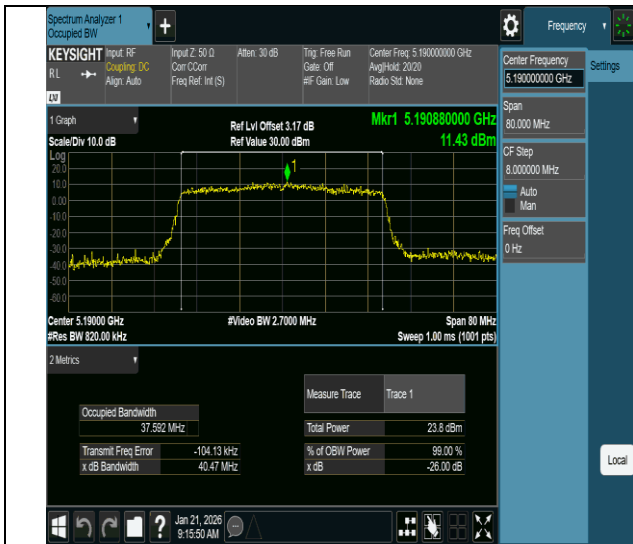
11ax40MIMO-Ant2-5190
