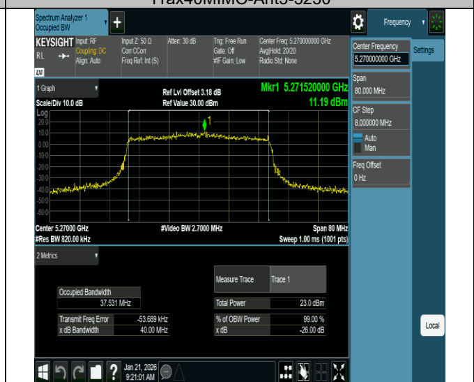
11ax40MIMO-Ant3-5270
