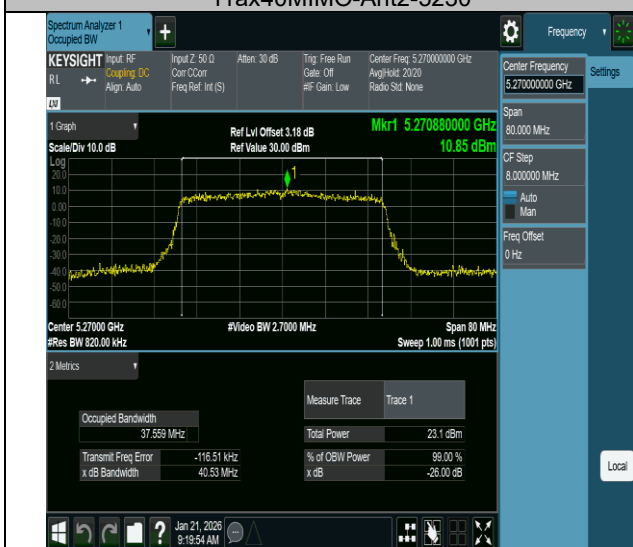
11ax40MIMO-Ant2-5270
