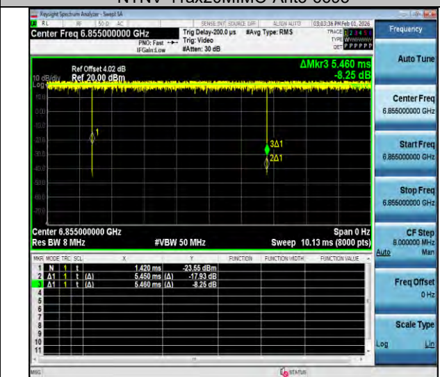
NTNV-11ax20MIMO-Ant3-6855
