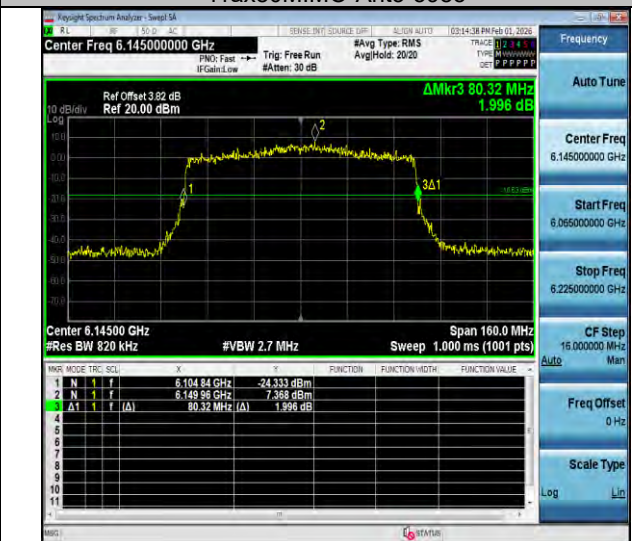
11ax80MIMO-Ant3-6145
