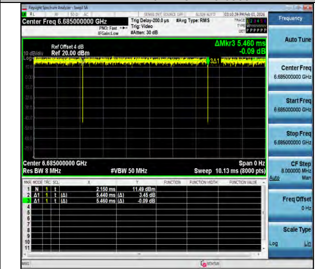
NTNV-11ax40MIMO-Ant3-6685
