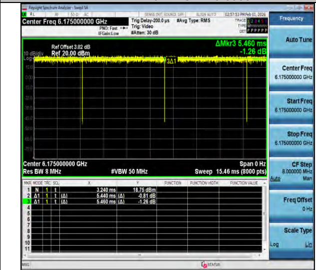
NTNV-11ax20MIMO-Ant3-6175
