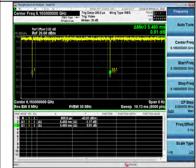
NTNV-11ax40MIMO-Ant3-6165
