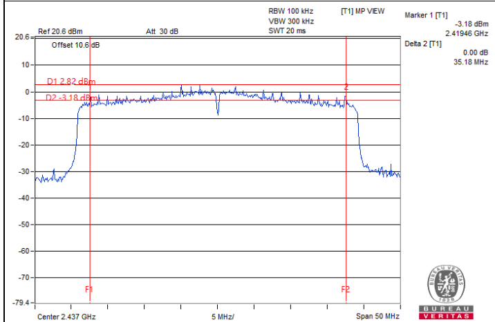
802.11ax (HE40) Full RU / Chain 1 : CH 6
