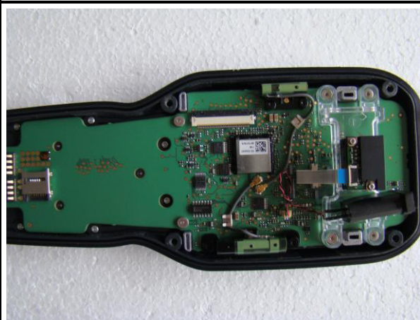
EUT OPEN TOP
