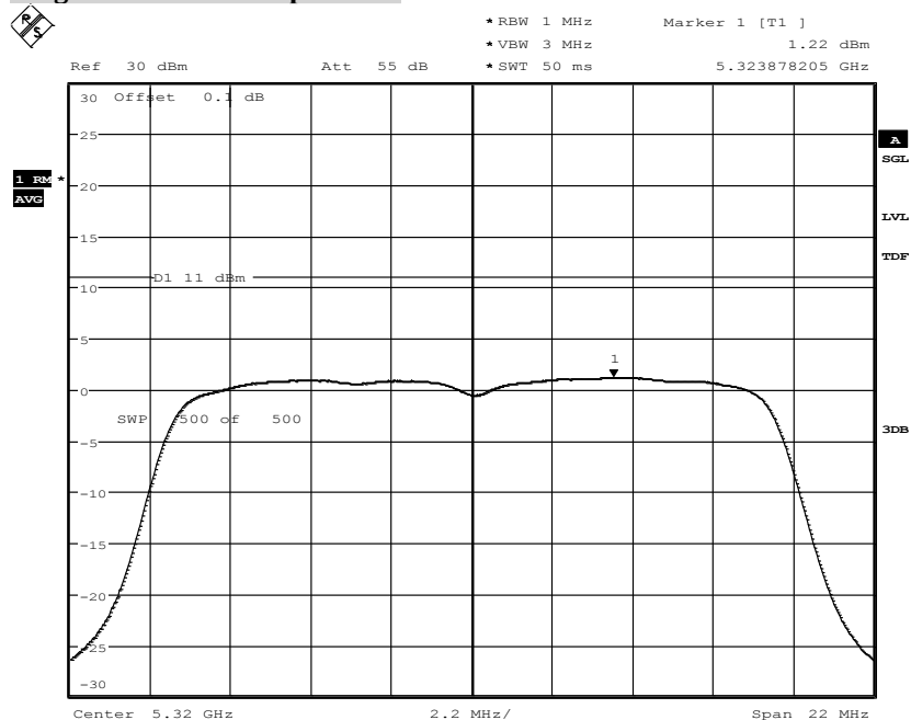
Diagram a-Mode 9Mbps Ch64:
