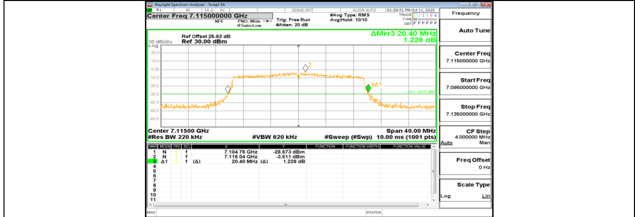
11AX20MIMO_Ant0_7115
