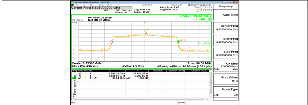
11AX40MIMO_Ant0_6525
