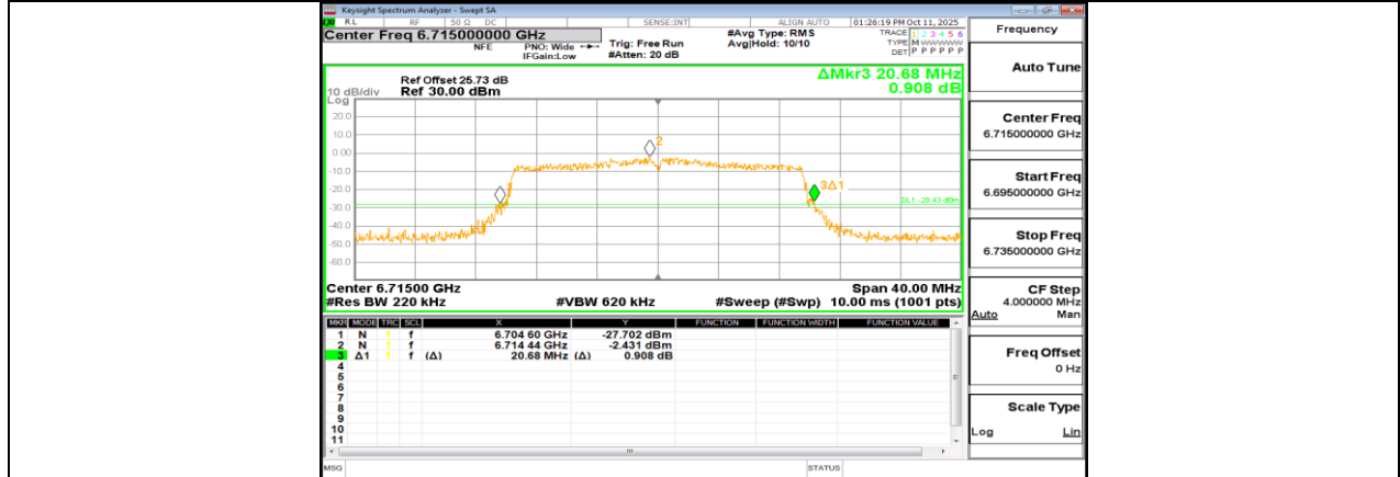
11AX20MIMO_Ant0_6715
