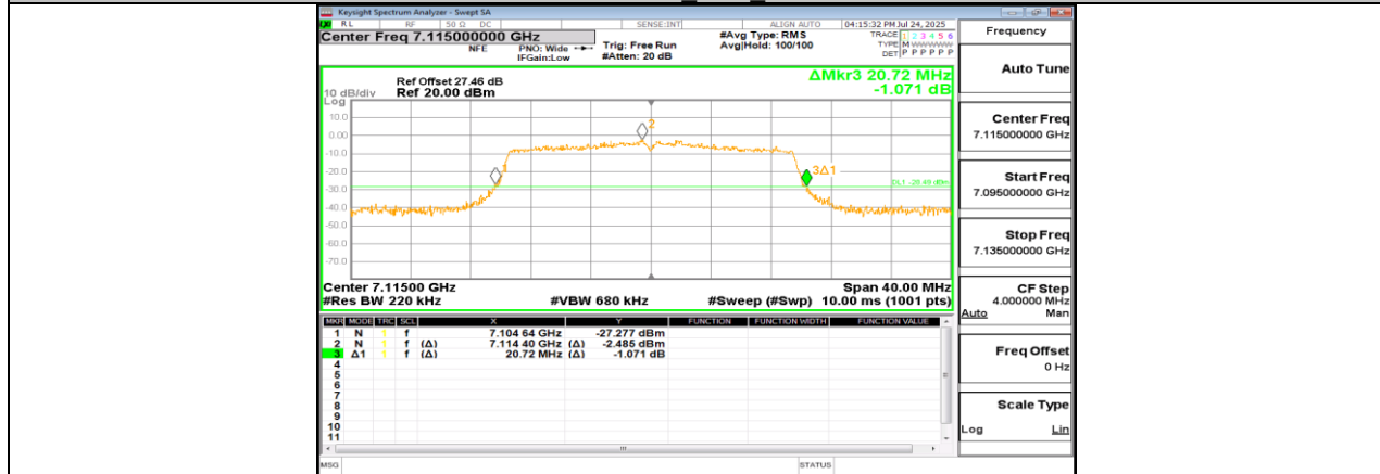
11A-CDD Ant1 7115
