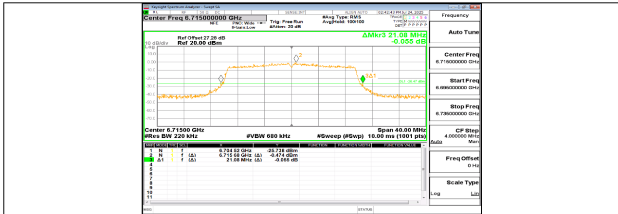
11A-CDD Ant1 6715
