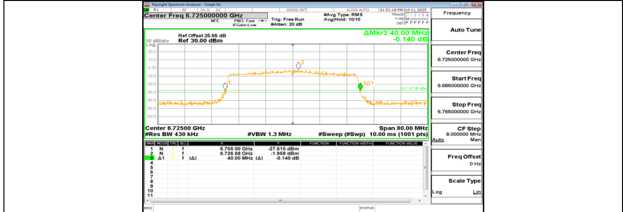
11AX40MIMO_Ant0_6725
