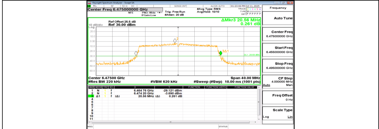
11AX20MIMO_Ant0_6475
