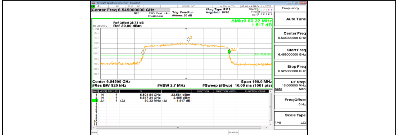
11AX80MIMO_Ant0_6545
