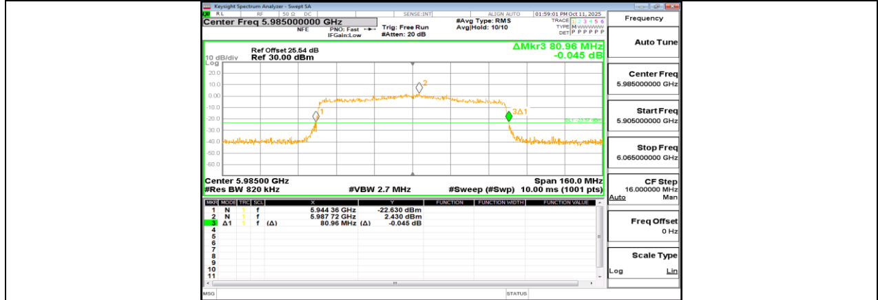
11AX80MIMO_Ant1_5985
