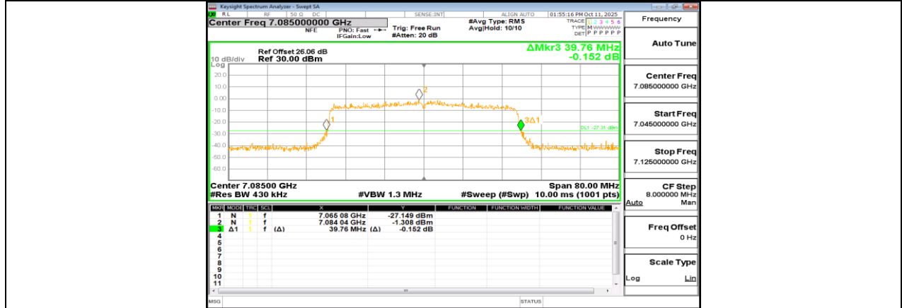
11AX40MIMO_Ant0_7085
