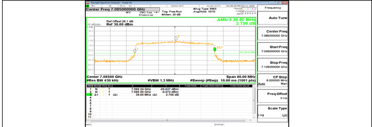
11AX40MIMO_Ant1_7085
