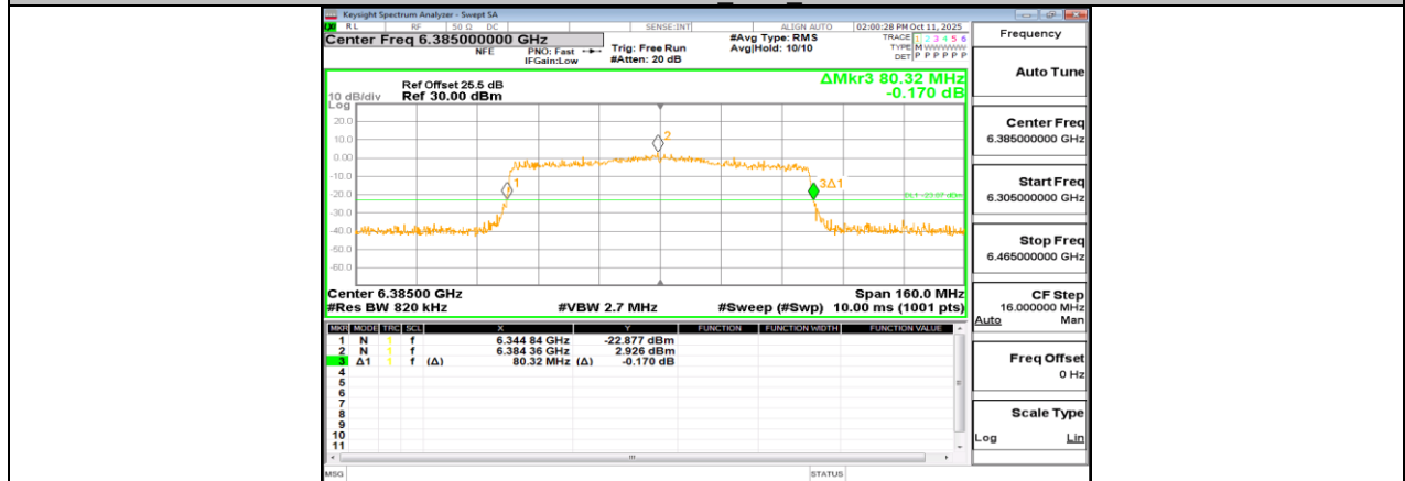
11AX80MIMO_Ant1_6385
