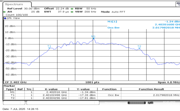
BLE_2M_Ant0_2402
