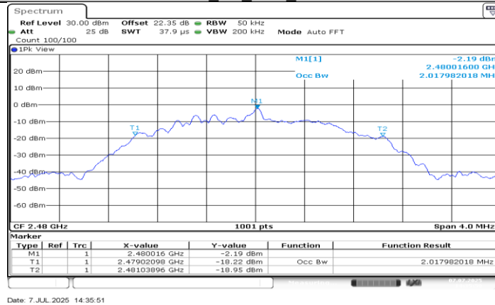
BLE_2M_Ant0_2480
