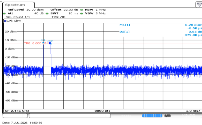
3DH1_Ant0_Hop
