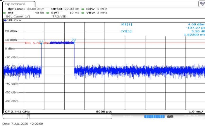
3DH3_Ant0_Hop
