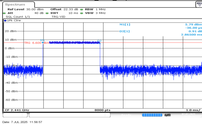
3DH5_Ant0_Hop
