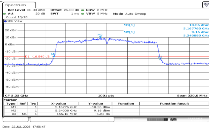
11AC160MIMO_Ant1_5250
