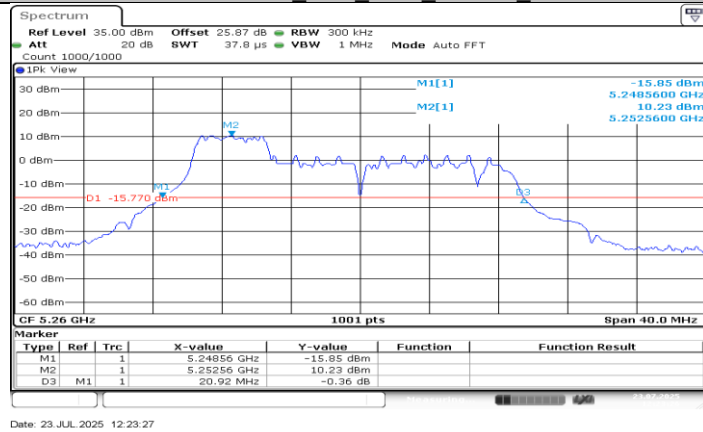
11AX20MIMO_Ant1_5260_52Tone_RU37
