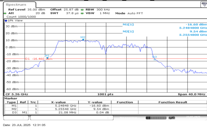
11AX20MIMO_Ant1_5260_106Tone_RU53
