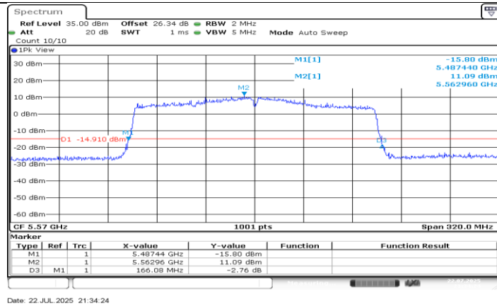
11AX160MIMO_Ant0_5570
