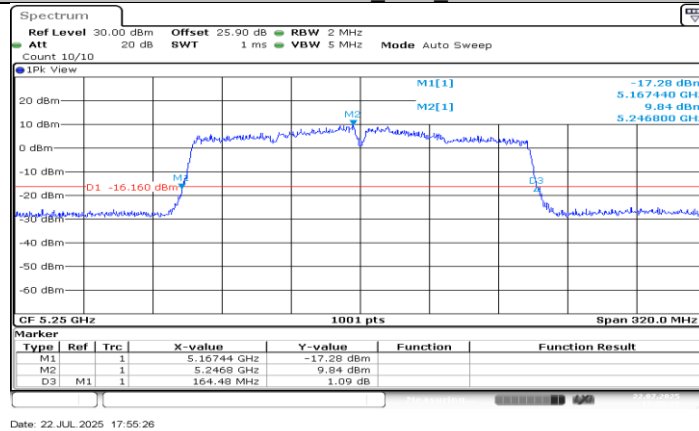
11AC160MIMO_Ant0_5250
