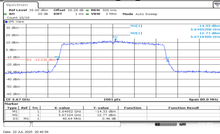
11AX40MIMO_Ant0_5670
