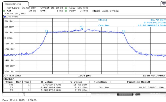
11AX20MIMO_Ant0_5500
