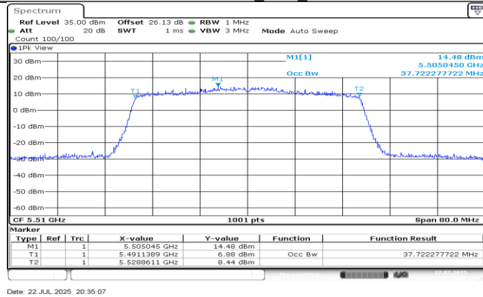
11AX40MIMO_Ant0_5510
