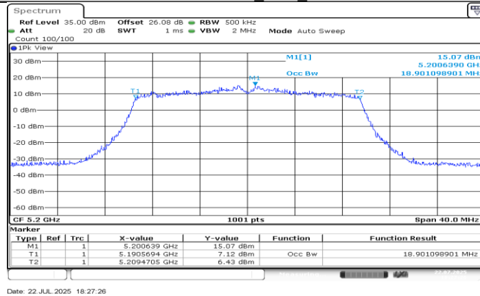
11AX20MIMO_Ant0_5200
