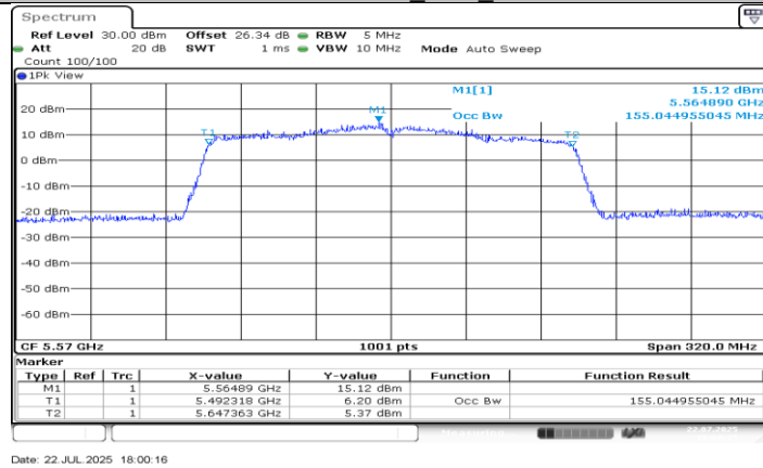
11AC160MIMO_Ant0_5570
