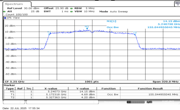
11AC160MIMO_Ant0_5250
