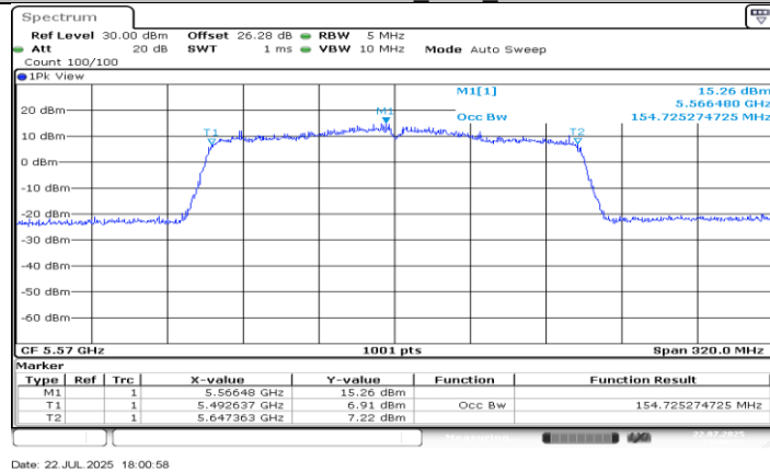
11AC160MIMO_Ant1_5570
