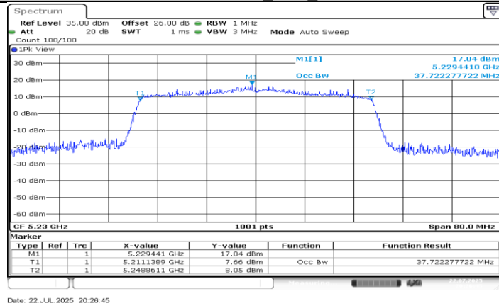
11AX40MIMO_Ant0_5230
