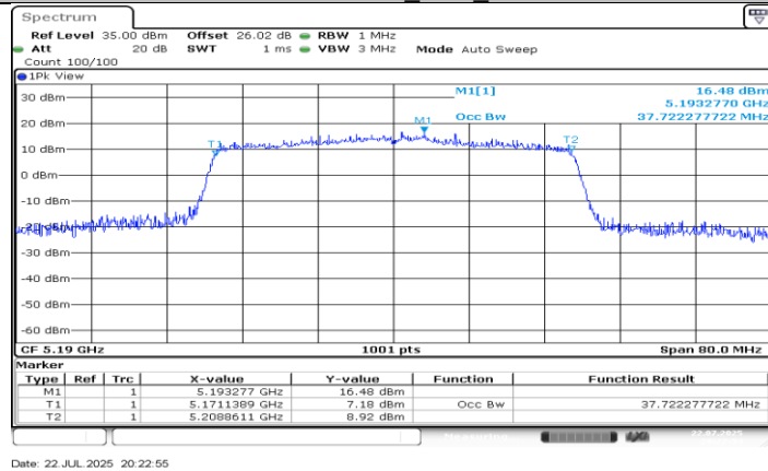
11AX40MIMO_Ant0_5190
