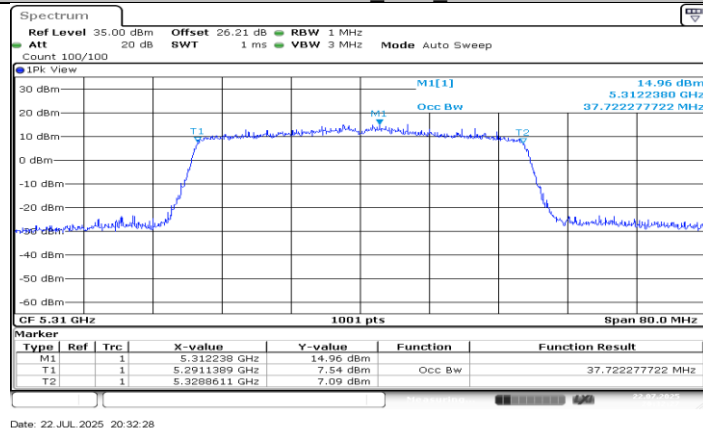
11AX40MIMO_Ant0_5310
