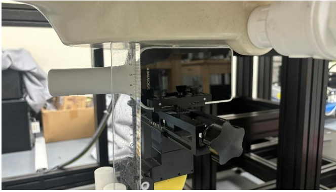
Right Edge(0mm)
