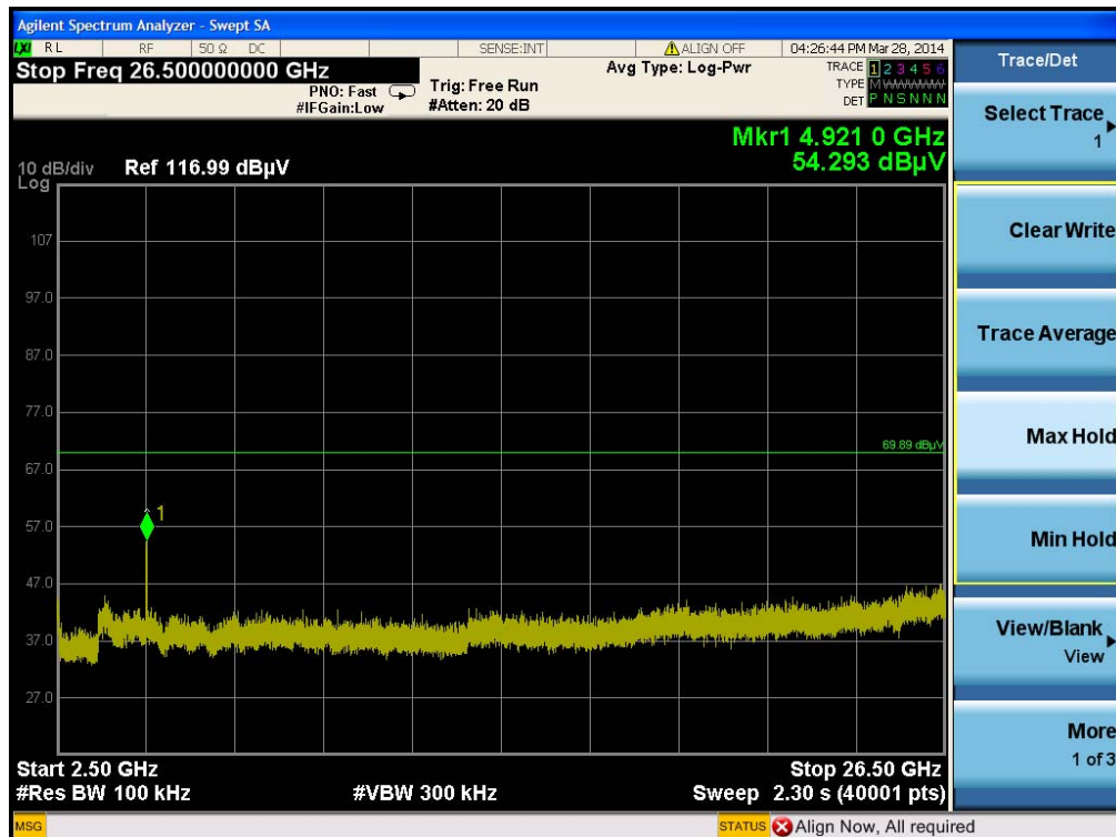
Plot on Configuration IEEE 802.11n MCS0 HT20 / CH 11 / 2500MHz~26500MHz (down 30dBc)
