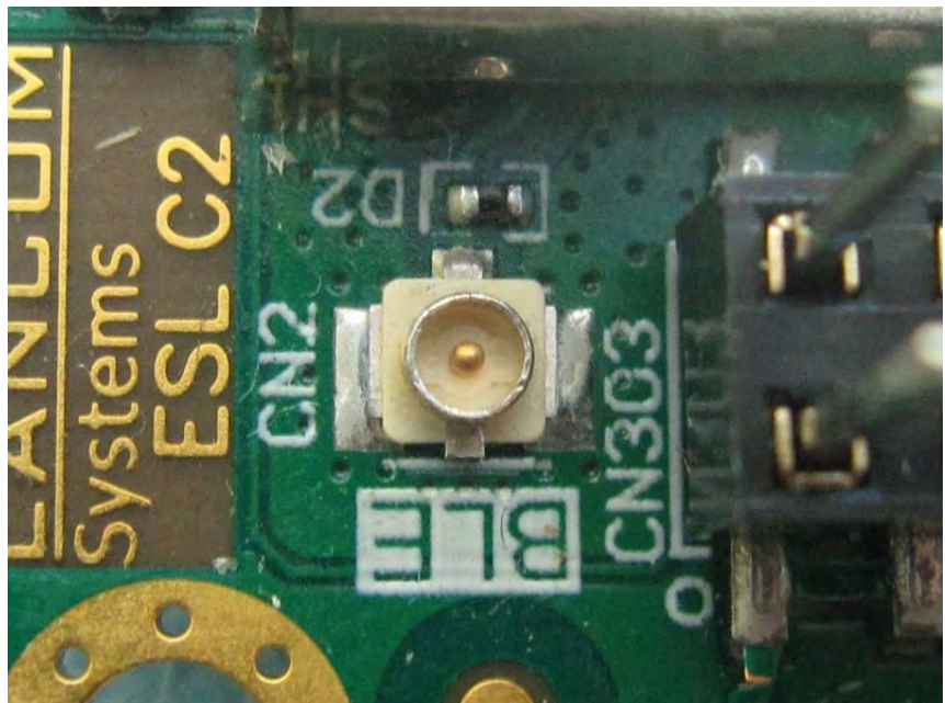
BLE connector
