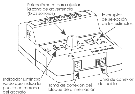
Esquema n° 1: caja emisora
