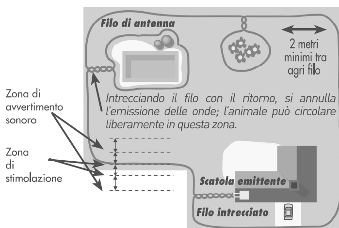
Schema n°4: esempio di installazione
