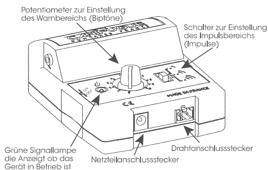
Schema Nr. 1: Sender
