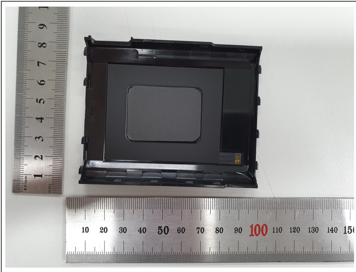
<NFC Antenna>
