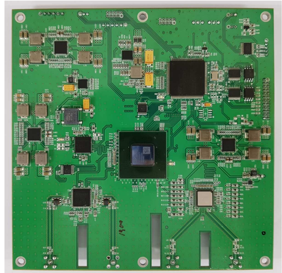
Bottom Layer
