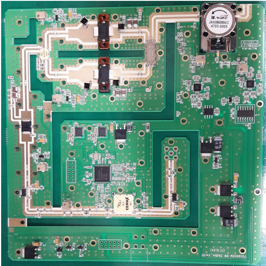
Top Layer
