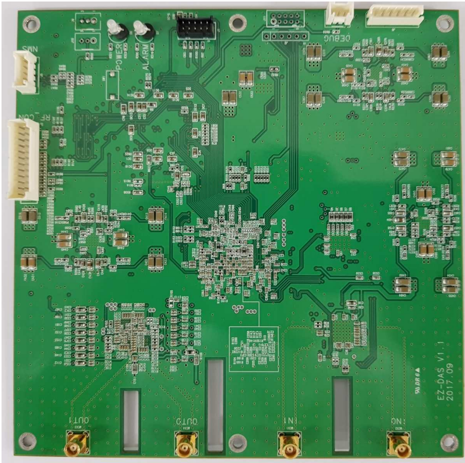
Top Layer
