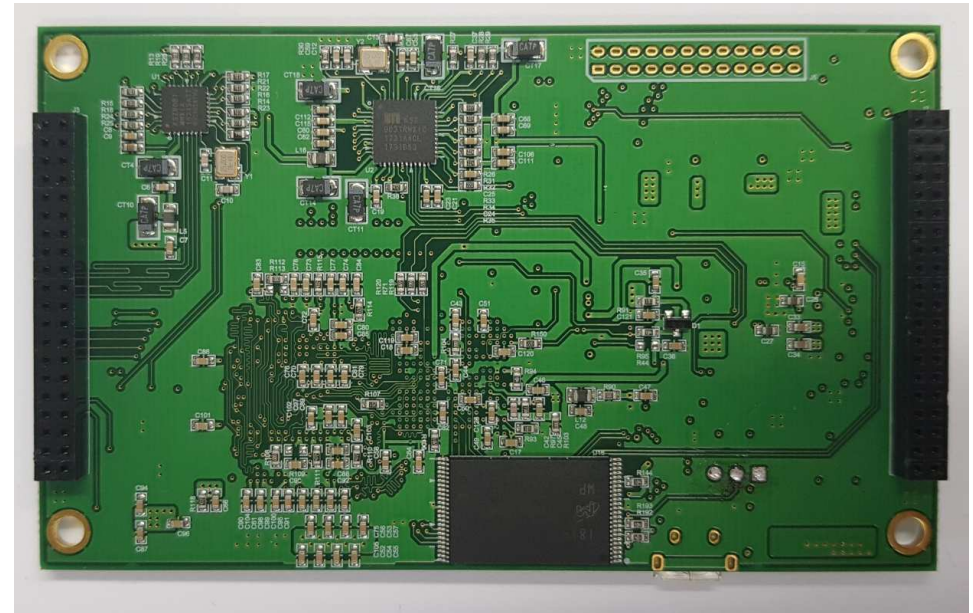
Bottom Layer
