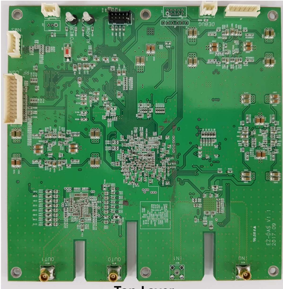
Top Layer
