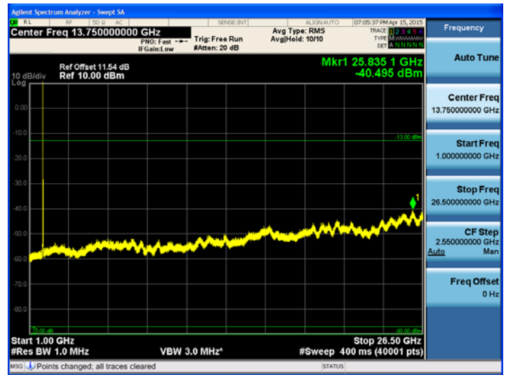
1900 MHz band ( 1 GHz – 26.5 GHz) CDMA Mid
