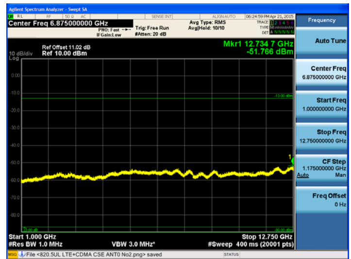
800 MHz band (1 GHz – 12.75 GHz)CDMA+LTE 5MHz
