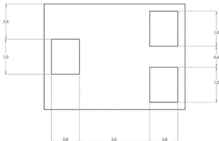
Bottom Side
