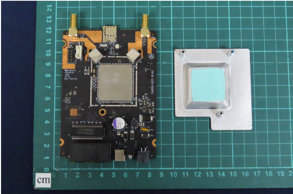
(3) EUT Photo
