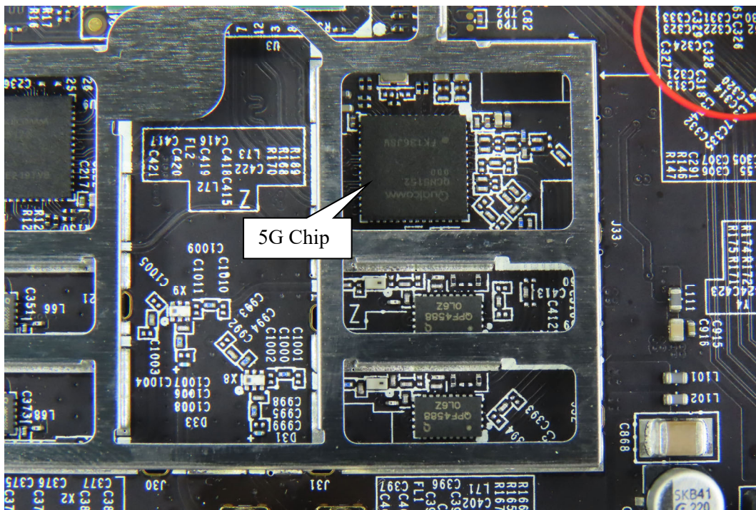
(13) EUT Photo
