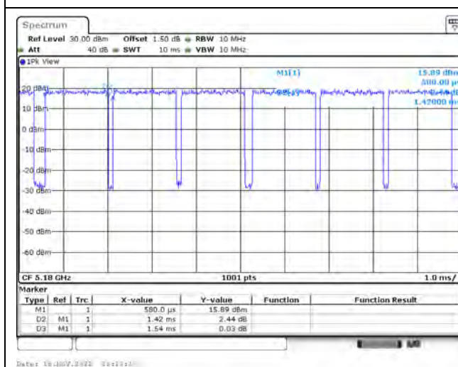
802.11a
