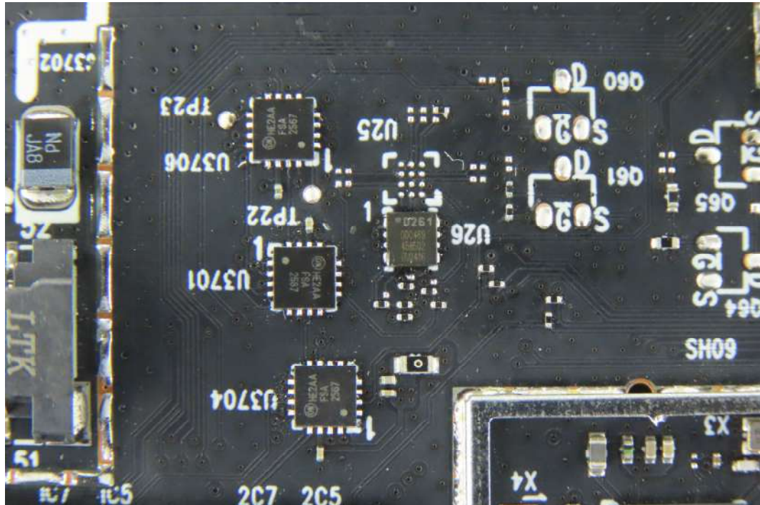
(15) EUT Photo_eSIM : MFXS-M006B-MFOCMW
