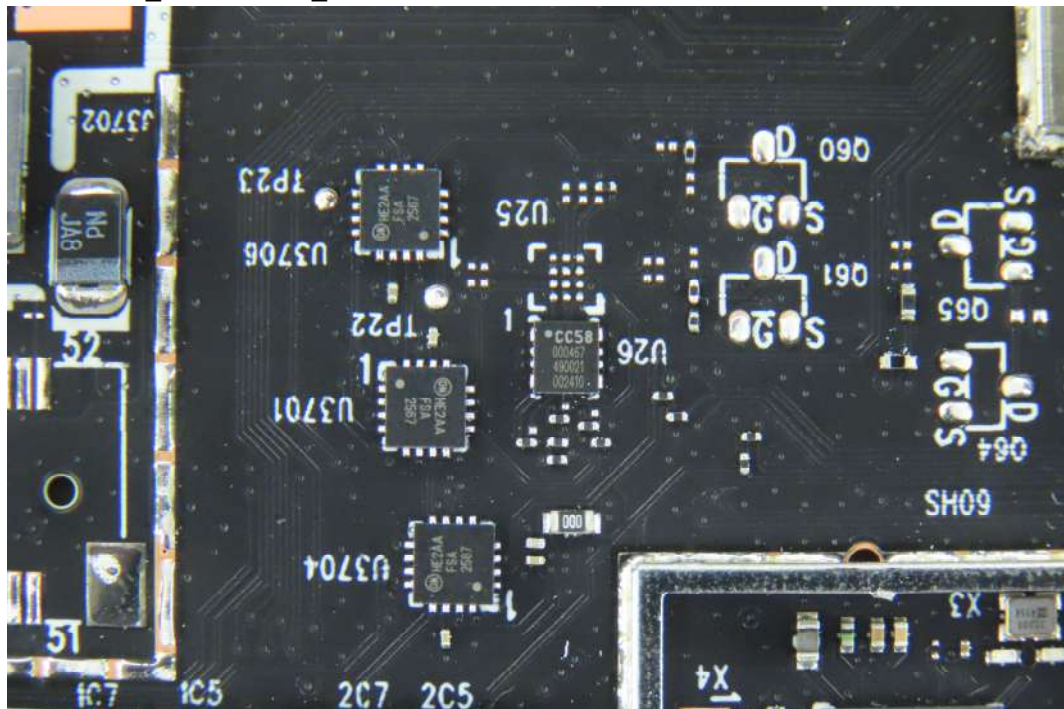
(16) EUT Photo_eSIM : eSIM_MFXS-A028a-MFOCMW
