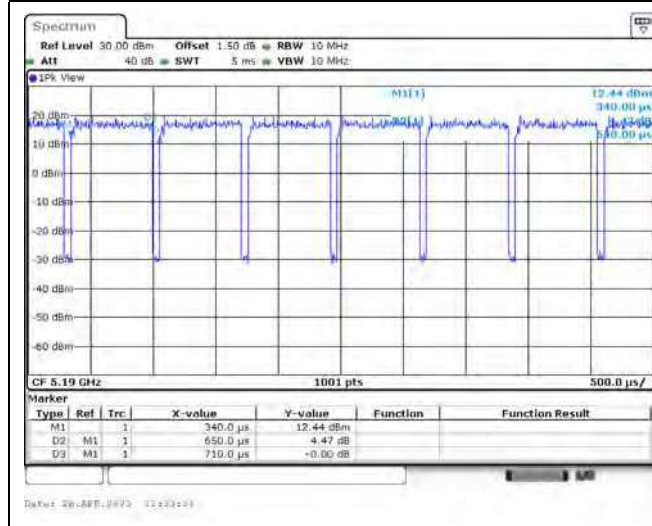
802.11ac (40 MHz)
