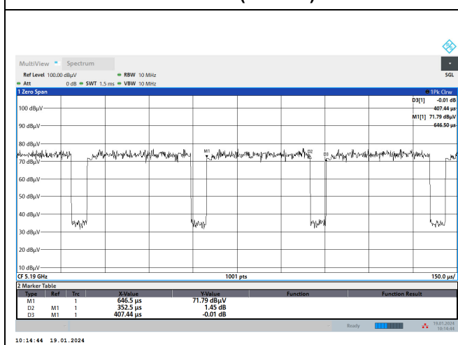
802.11ac (40 MHz)
