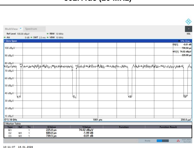
802.11ac (20 MHz)
