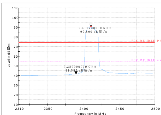
AV detector
