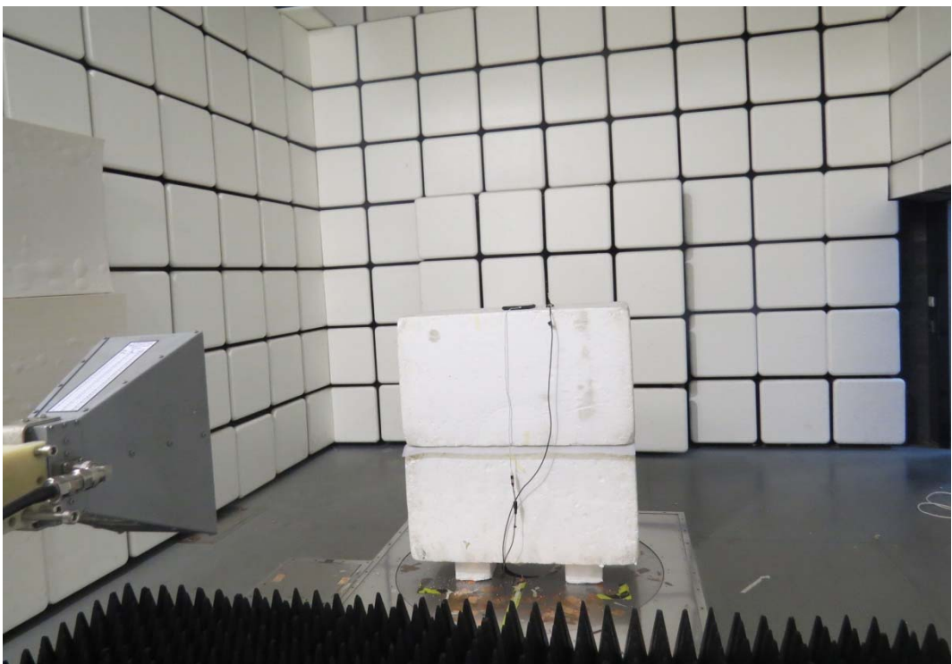
1GHz-18GHz
